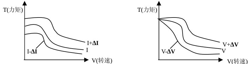
图 6. 矩频特性图
