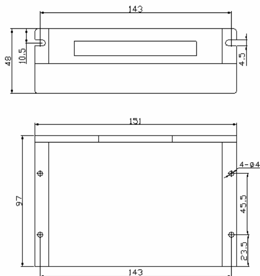
图 1. 安装尺寸图
