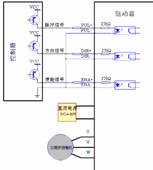
图 8. 3ND883 配三相混合式步进电机接线
