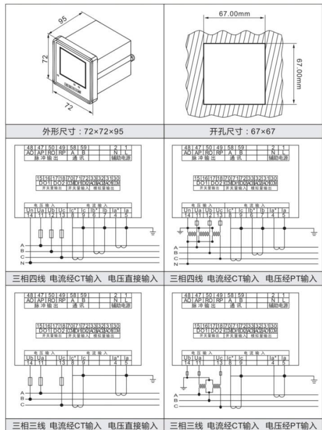
■ 72型(外形尺寸: 72×72×95 mm 开孔尺寸: 67.00×67.00mm)
