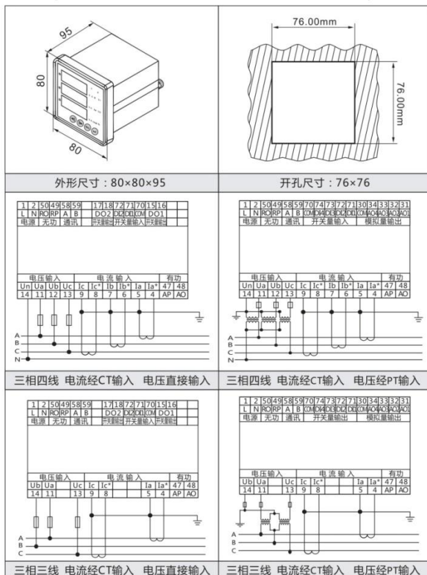
■ 80型(外形尺寸: 80×80×95 mm 开孔尺寸: 76.00×76.00mm)
