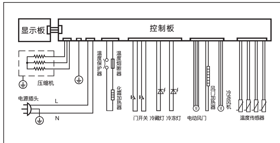
电路图
