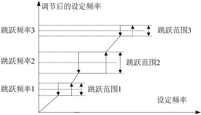
图 6-10 跳跃频率设定
