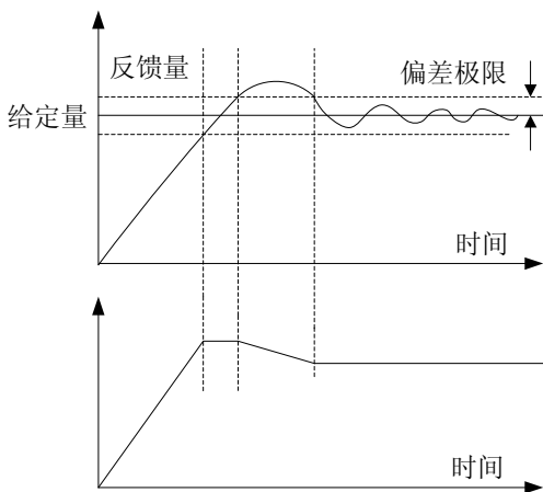
图 6-23 偏差极限示意图
