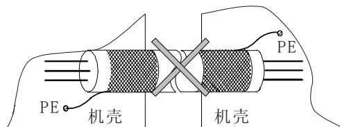
图 3-28 错误的屏蔽接地方法
