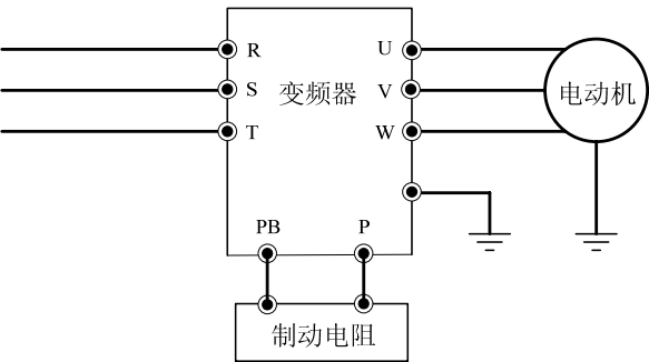
图 2-3 变频器与制动组件连线图（380V 18.5KW 以下）
