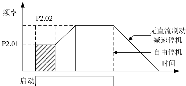
图 6-6 起动与停机频率输出曲线
