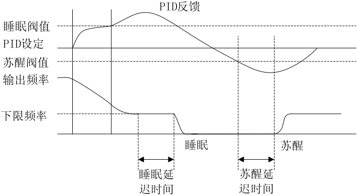
图 6-25 睡眠与苏醒功能示意图
