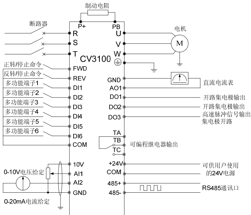
图 3—17 基本运行配线图
