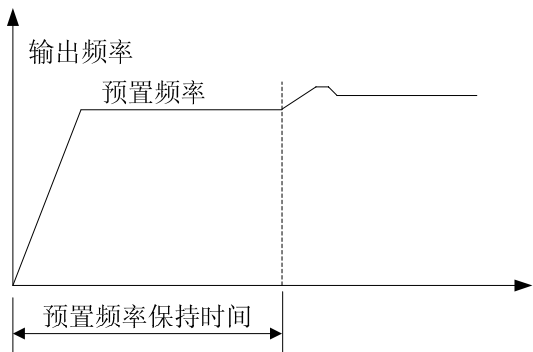
图 6-24 闭环预置频率运行示意图
