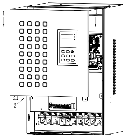
图 3-10 盖板的安装
