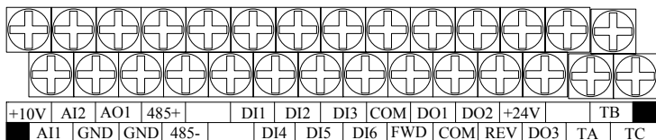
图 3-19 控制板端子排列顺序图 (11KW-18.5KW 控制板)
