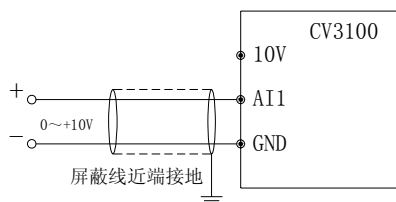
图 3-21 AI1 端子配线图
