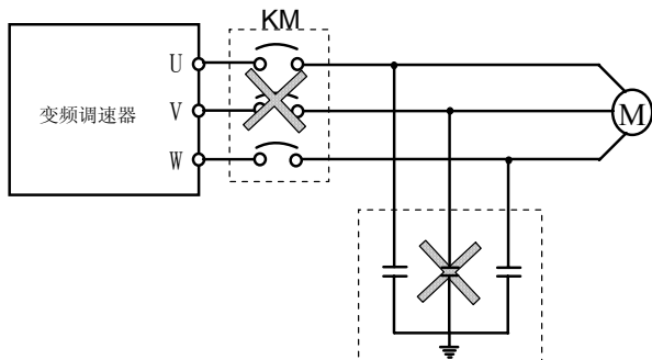
图 1-3 变频器输出端禁止使用电容器
