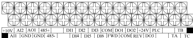
图 3-20 控制板端子排列顺序图 (22KW 以上控制板)
