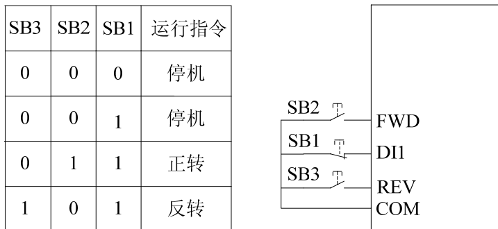
图 6-13 三线式控制模式 1
