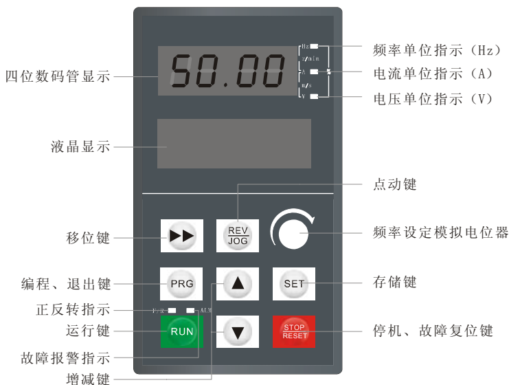
图 4-3 远控操作键盘示意图
