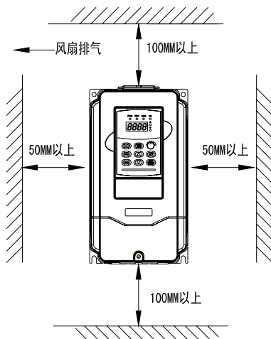
图 3-1 安装的间隔距离图
