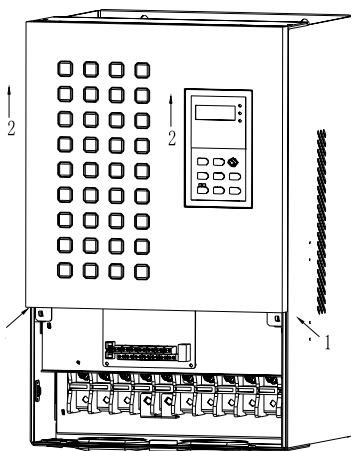
图 3-9 盖板的拆卸
