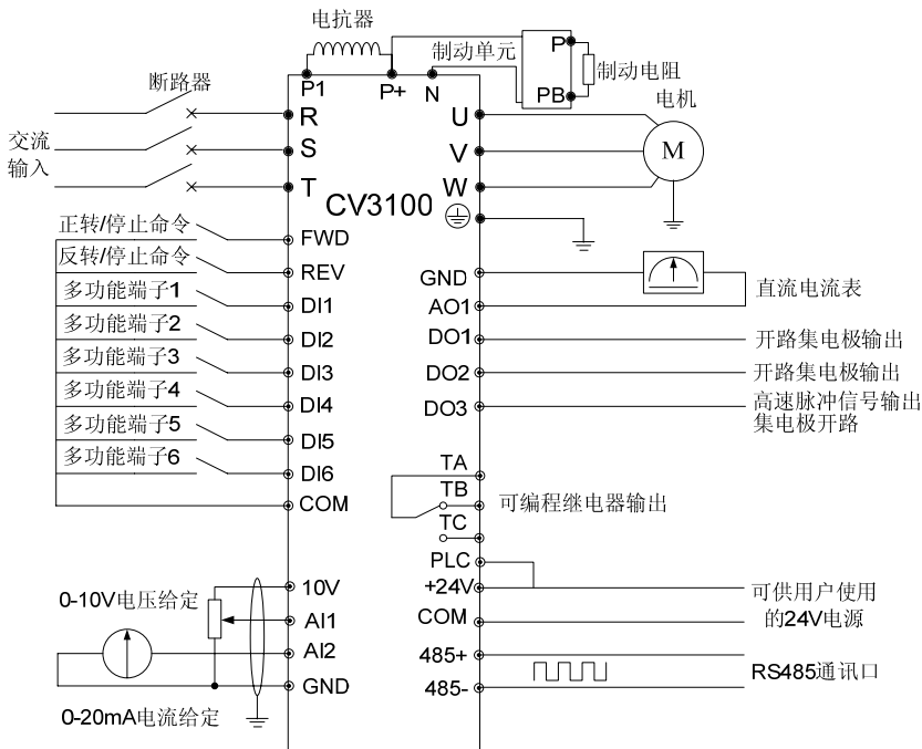
图 3-18 基本运行配线图
