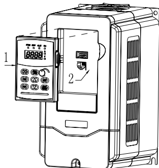
图 3-4 操作面板的安装
