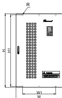
(c): 11KW~75KW 规格尺寸
