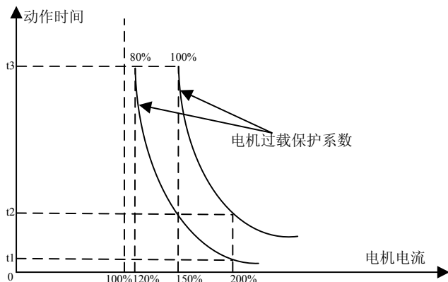
图 6-30 电机过载保护曲线示意图
