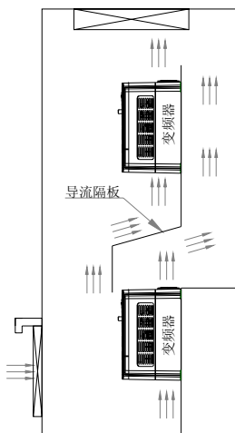
图 3-2 多台变频器的安装示意图
