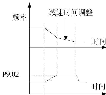
图 6-31 过压限制水平说明
