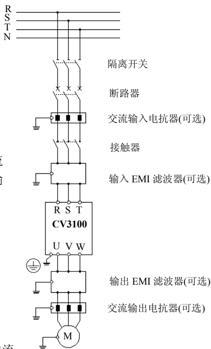
图 3-12 变频器与选配件的连接
