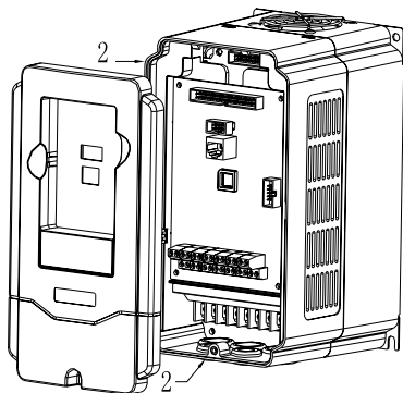
图 3-6 盖板的安装
