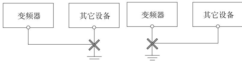
图 3-15 共用接地极示意图 (a)
