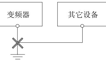
图 3-16 共用接地极示意图 (b)
