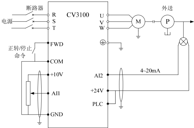
图 6-20 模拟反馈控制系统示意图
