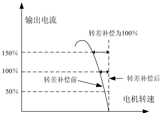
图 6-2 转差频率补偿说明
