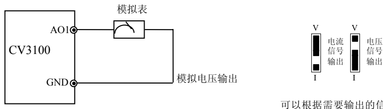
图 3-23 模拟输出端子配线
