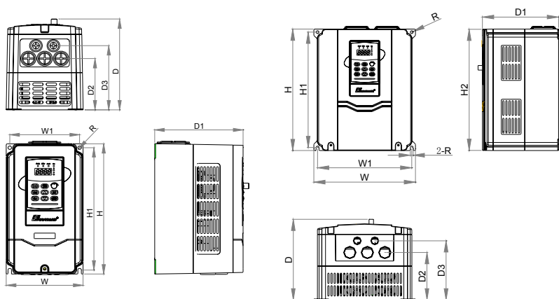
(a): 0.75KW~4.0KW 规格尺寸
