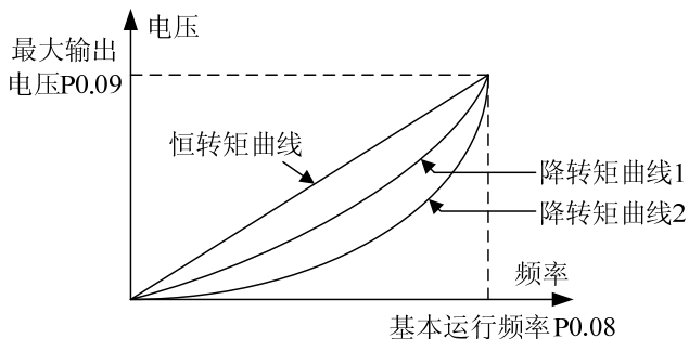
图 6-4 V/F 曲线
