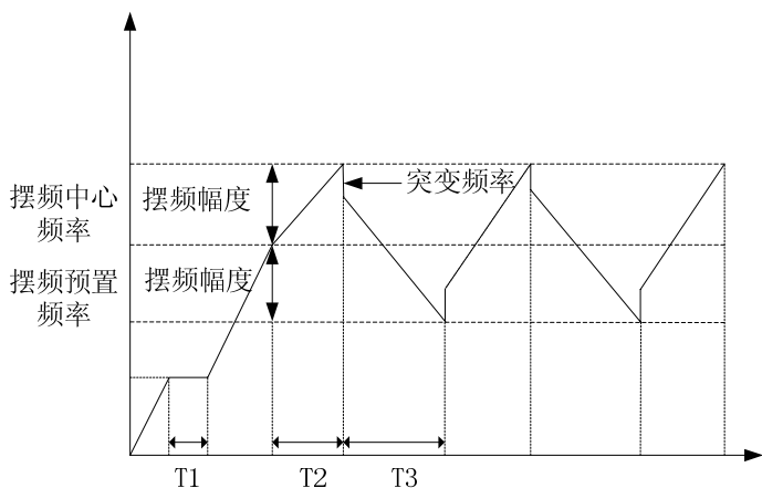
图 6-29 摆频设定说明
