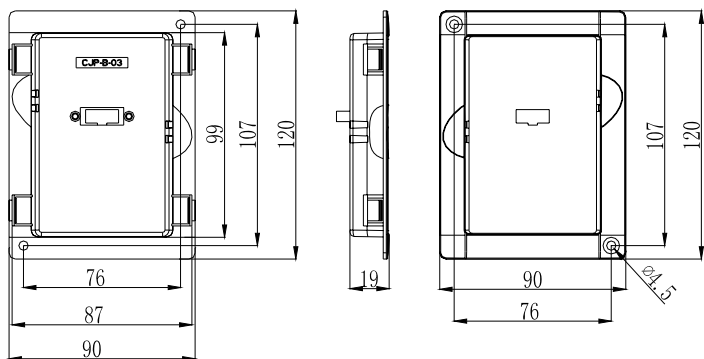
图 2-1 CV3100-LKD 外引托板尺寸（选配件）
