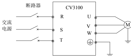
图 3-11 主回路简单配线
