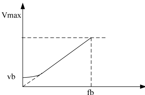
图 6-1 转矩提升设置
