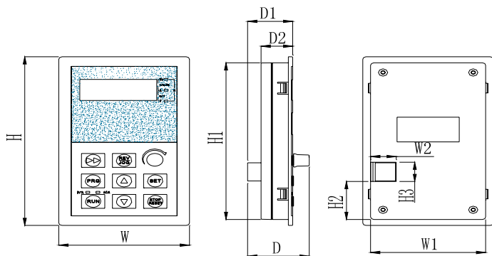
图 2-1 CV3100-LKD 外引托板尺寸（选配件）
