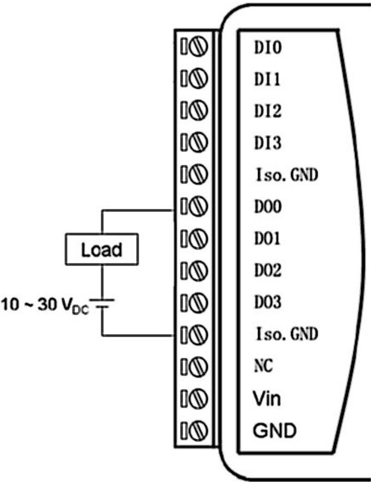
图 1.5 数字量输出接线
