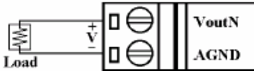
图 1.2 电压输出接线
