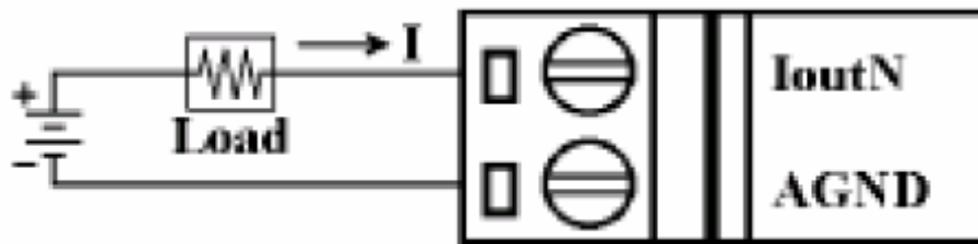
图 1.3 电流输出接线
