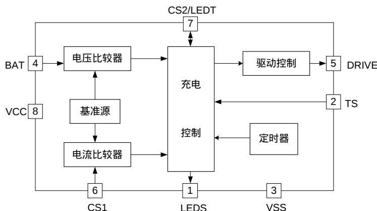
图 1 VM7205 功能框图
