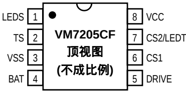
图 2 VM7205 引脚排列
