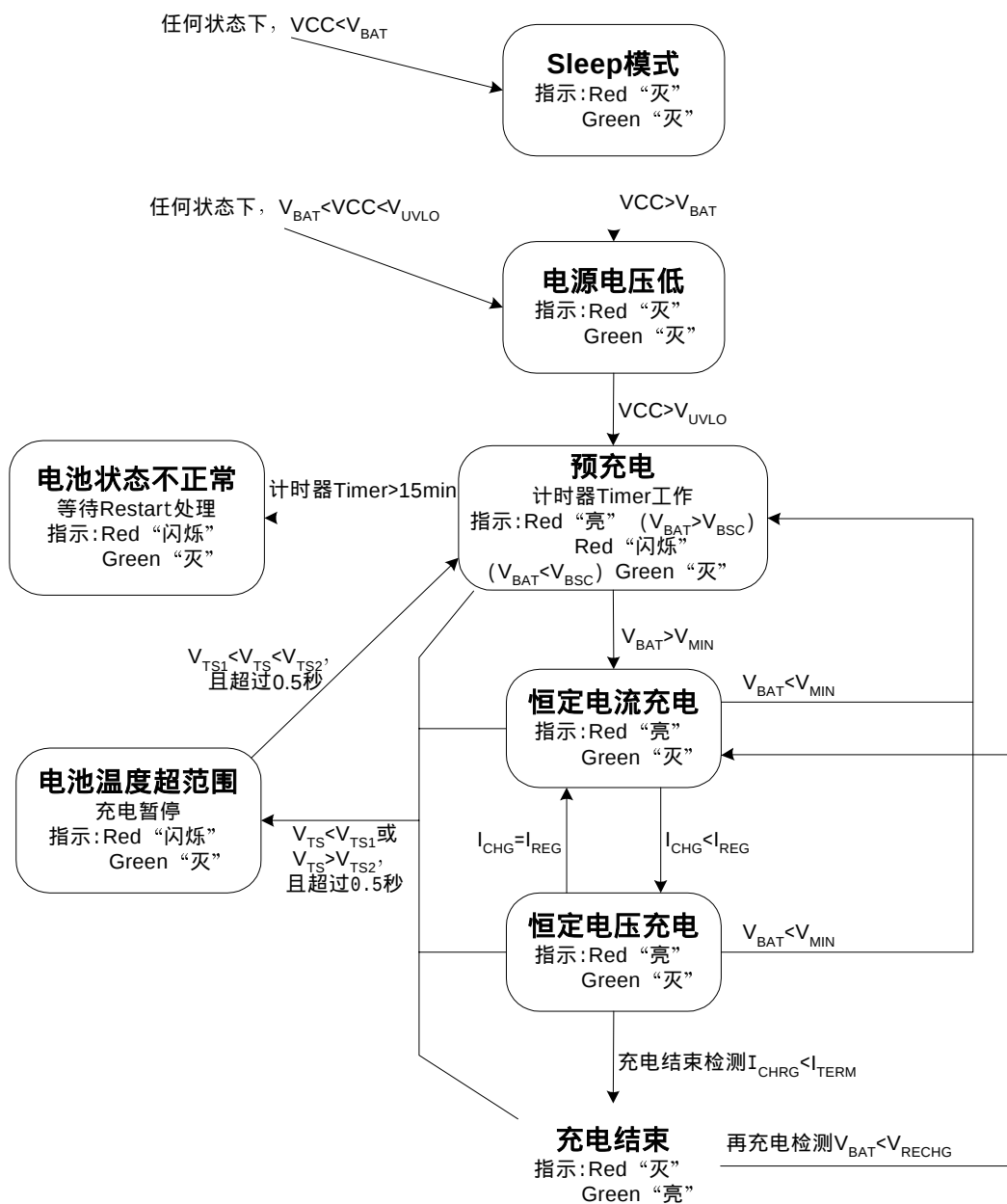
图 6 充电周期的流程图
