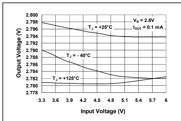
图 2-6: 输出电压—输入电压（ V_R = 2.8V ）曲线
