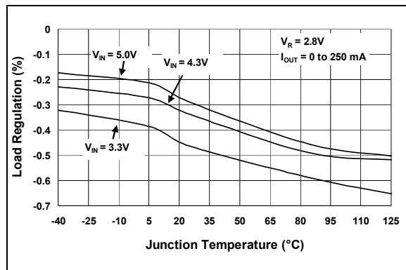
图 2-28：负载稳定度—结温 ( V_R = 2.8V ) 曲线
