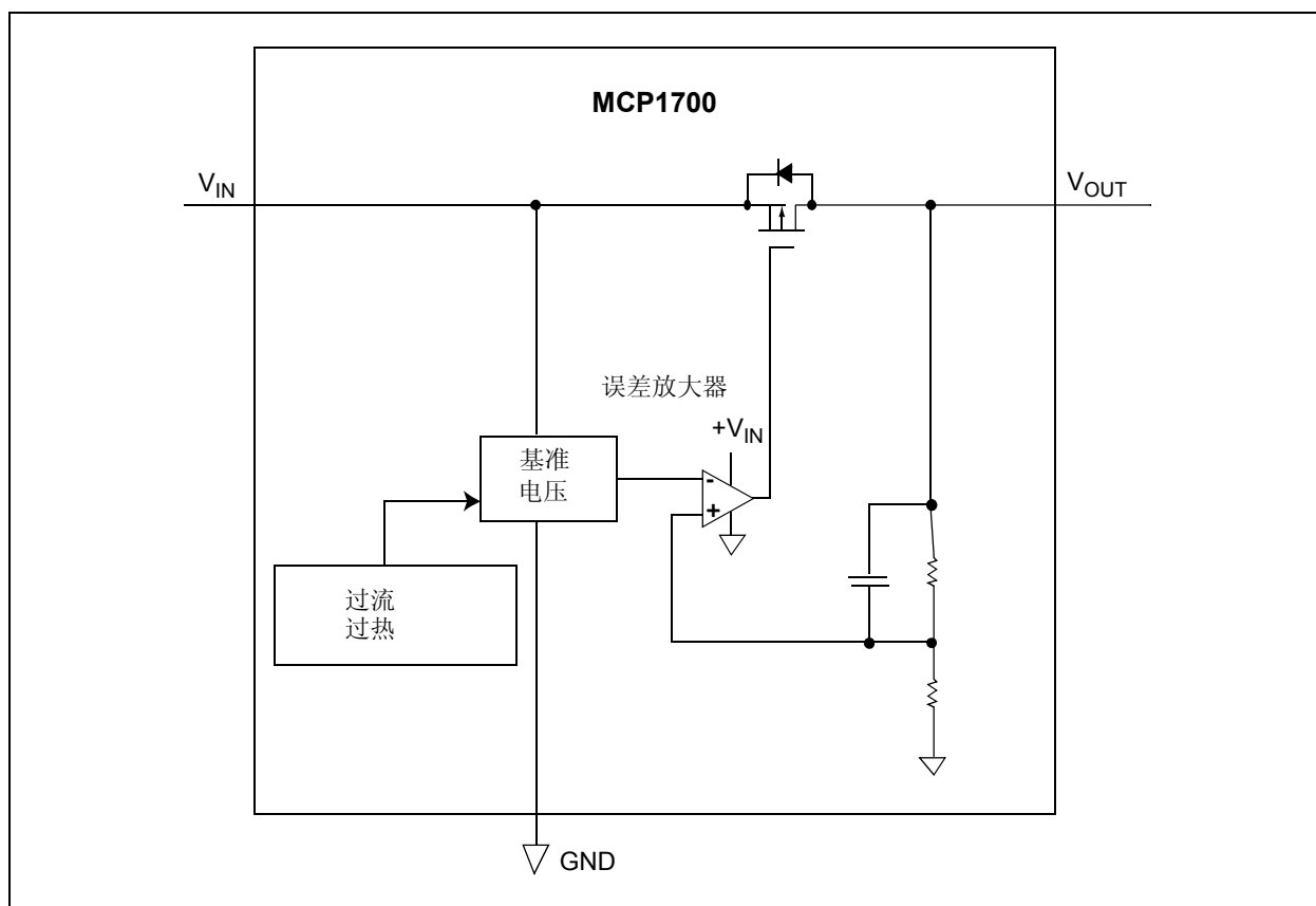
图 4-1: 结构框图
