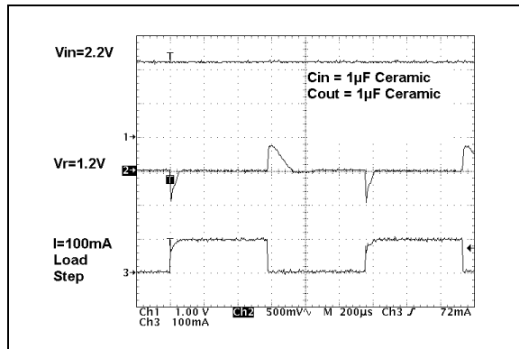
图 2-17: 动态负载响应 ( V_R = 1.2V )
