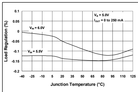
图 2-29：负载稳定度—结温 ( V_R = 5.0V ) 曲线
