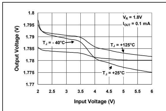
图 2-5: 输入电压—输入电压（ V_R = 1.8V ）曲线
