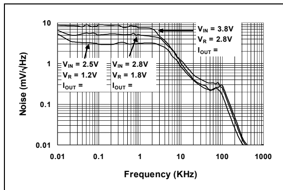
图 2-16: 噪声—频率曲线
