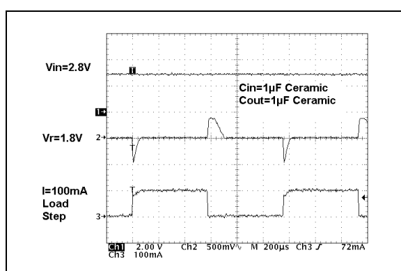
图 2-18: 动态负载响应 ( V_R = 1.8V )
