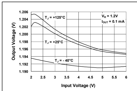
图 2-4: 输出电压—输入电压（ V_R = 1.2V ）曲线
