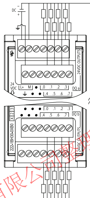
SM 1222 DQ 16 x 24 VDC
