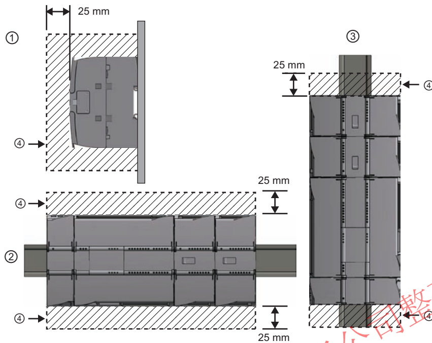
① 侧视图
