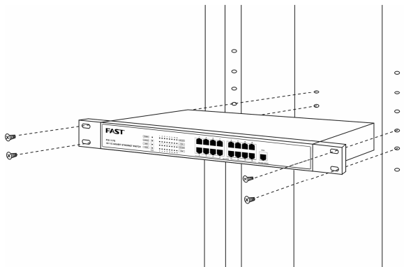
3.2 把交换机固定在支架上的示意图
