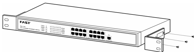
3.1 把 L 型支架安装到 FS117G 交换机上的示意图
