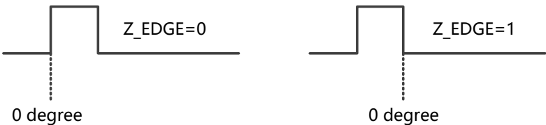
图-13: Z 脉冲的沿和零位的关系
