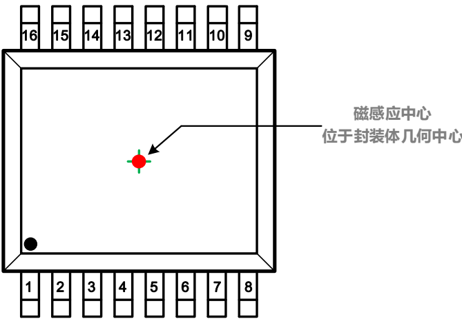
图-1: MT6835 TSSOP-16封装外观图
