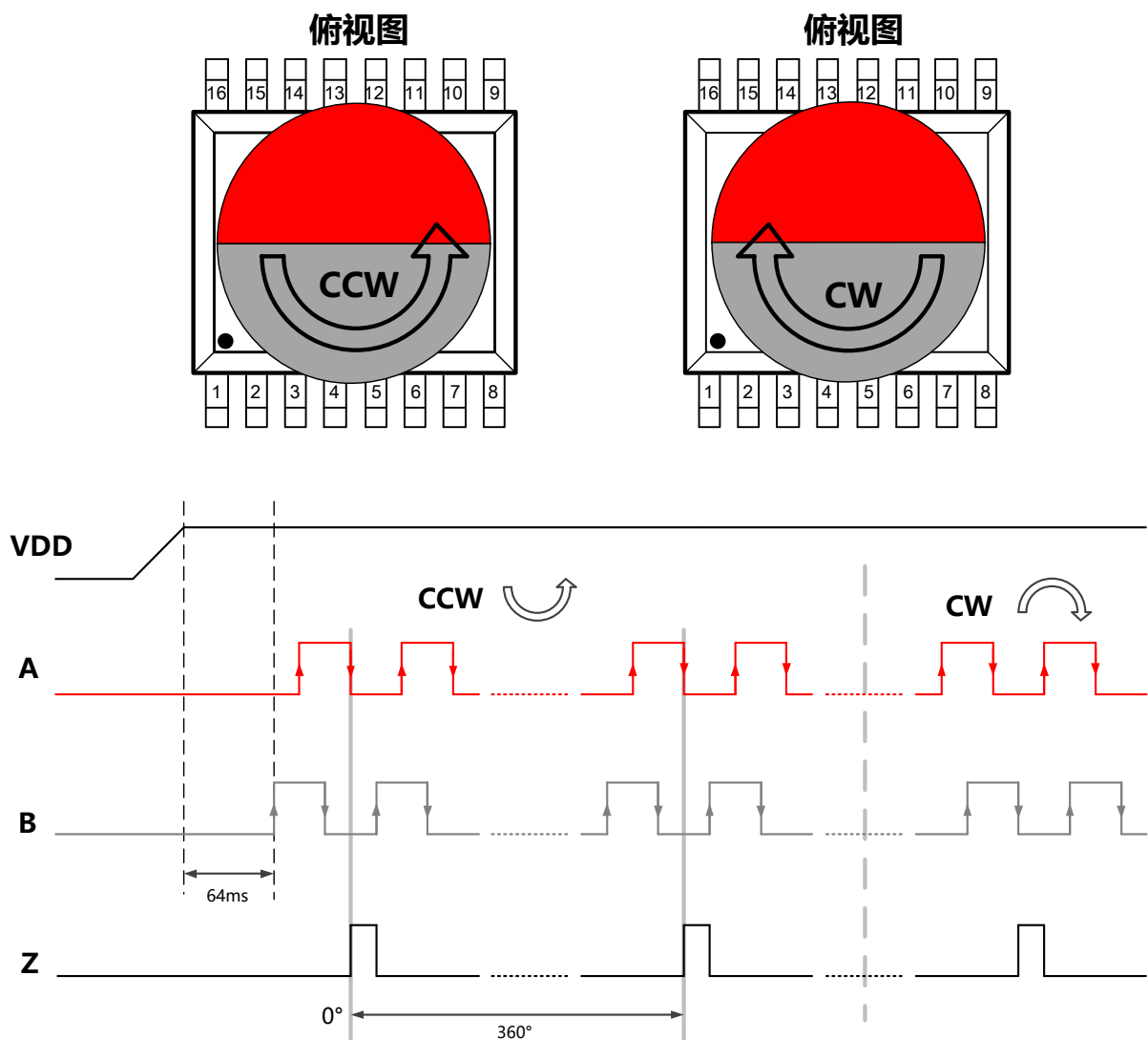
图-7: ABZ输出模式
