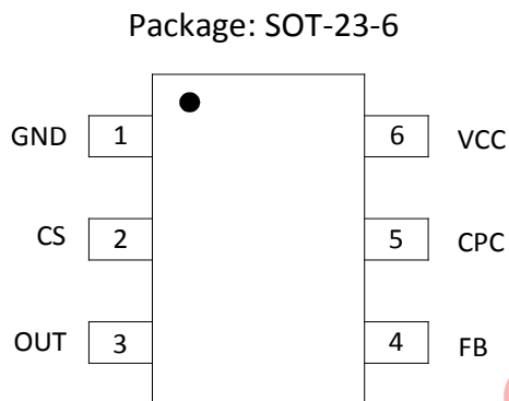
图 2. 管脚排布
