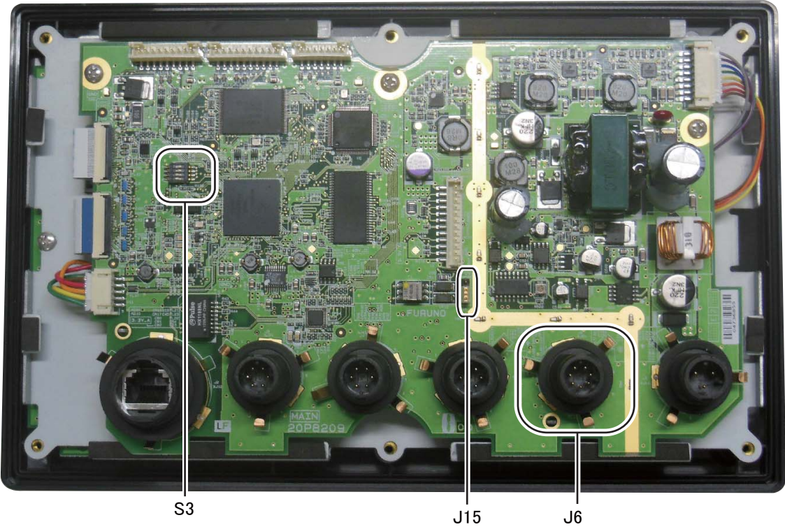
主板 20P8209
