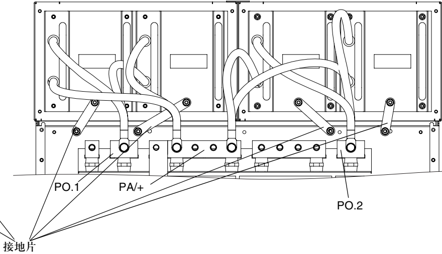
示例 4：ATV61H C50N4 ... C63N4
