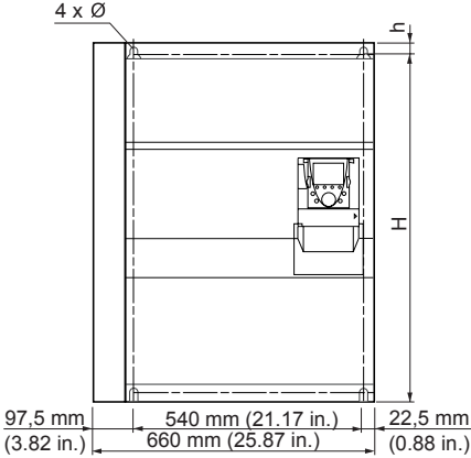
ATV61H C25N4D 至 C31N4D 带有制动单元 (VW3A7 101)
