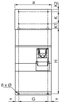
ATV61H C11Y 至 C20Y
