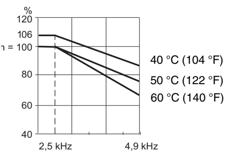
ATV61HC16Y
