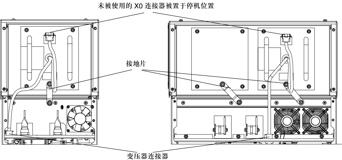
示例 1： ATV61H C11Y ... C20Y
