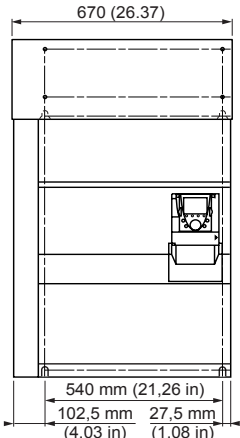
ATV61H C25Y 至 C40Y 带有制动单元
