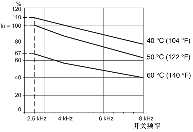
ATV61HD90N4
