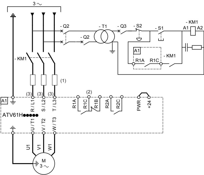
带有线路接触器的连接图
