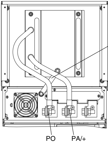
示例 1： ATV61H D55M3X ... D90M3X, ATV61H D90N4 ... C16N4
