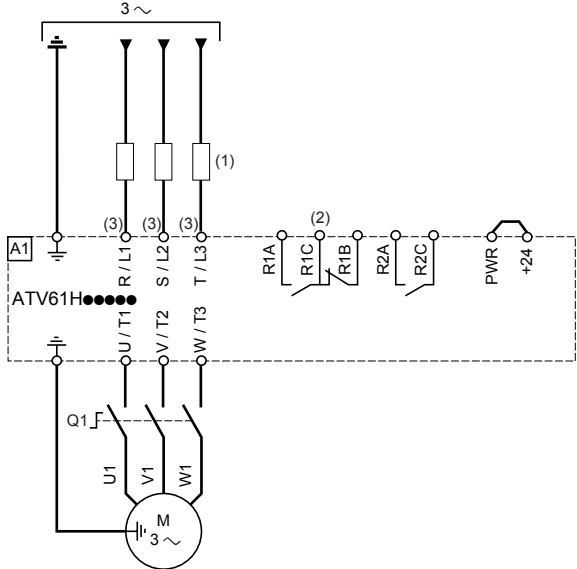
带有负荷开关的连接图
