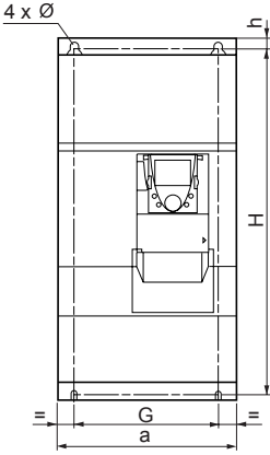
ATV61H D55M3XD 至 D90M3XD ATV61H D90N4D 至 C22N4D
