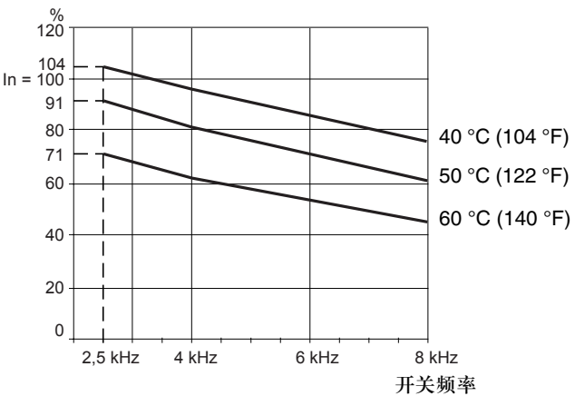
ATV61HC13N4
