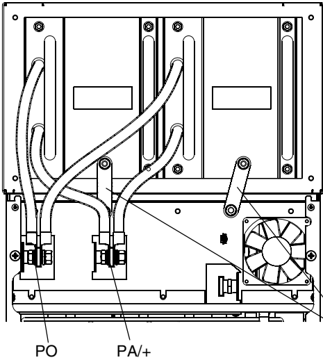
示例 2：ATV61H C22N4 ... C31N4
