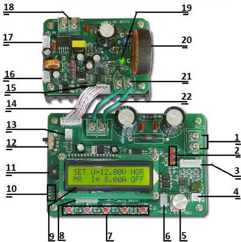
图 2-1 ZXY-6010S 面板
