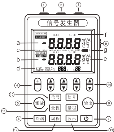
图 1 信号发生器正视图
