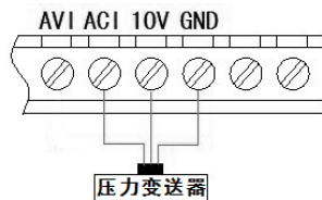
三线制压力变送器接线图
