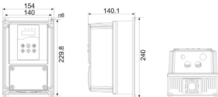
0.75-2.2kW 外型尺寸及安装尺寸示意图
