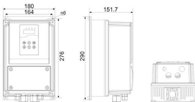
4-7.5kW 外型尺寸及安装示意图
