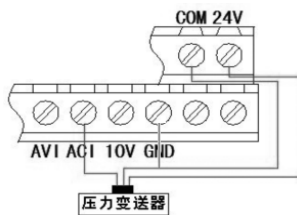
三线制压力变送器接线图
