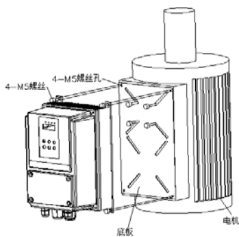
第三步：将变频器固定在铁板上
