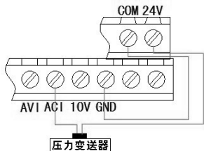
二线制压力变送器接线图
