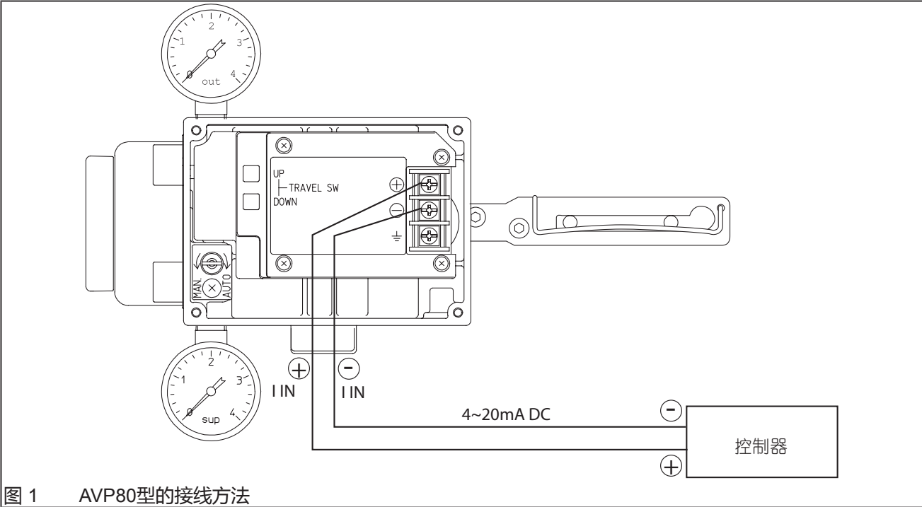
图 1 说明了AVP80 型（智能定位器）的接线方法。
