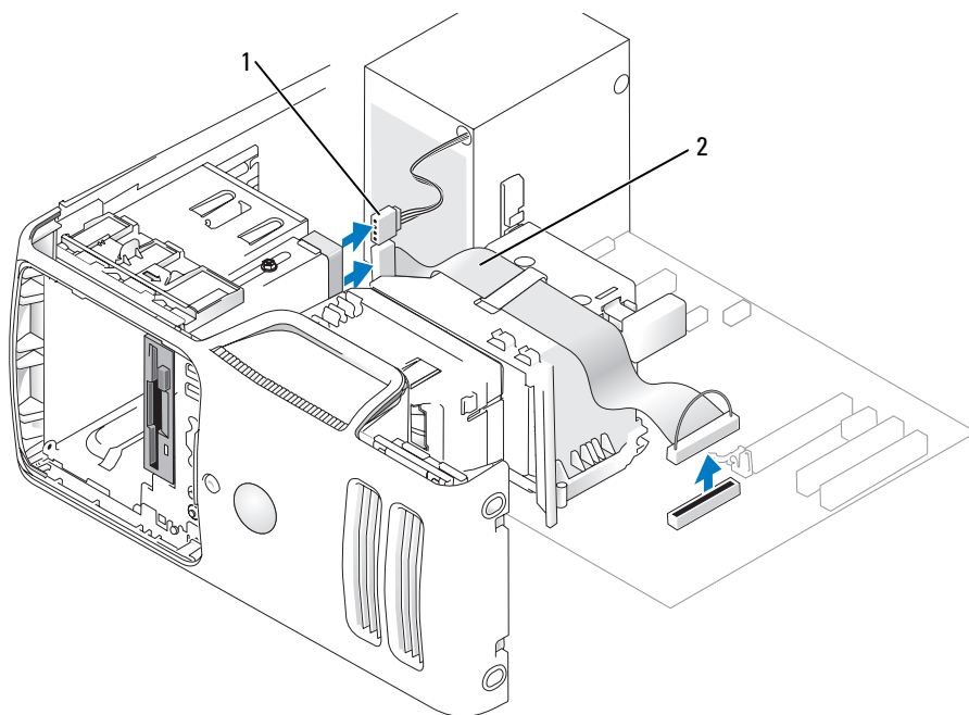
1 电源电缆
