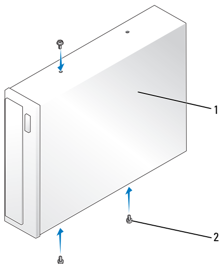
1 CD/DVD 驱动器
