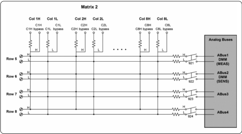
图 1. L4433A 双 / 四 4 × 8 干簧矩阵
