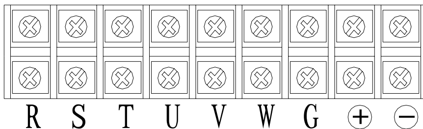
93KW 及以上标准品主回路端子 (220KW 及以上内置电抗器)
