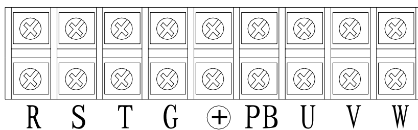
18.5~75KW 带制动单元主回路端子
