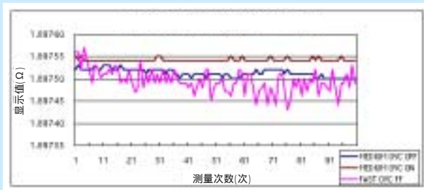
[低电能欧姆: 2 Ω 量程/快·中]
