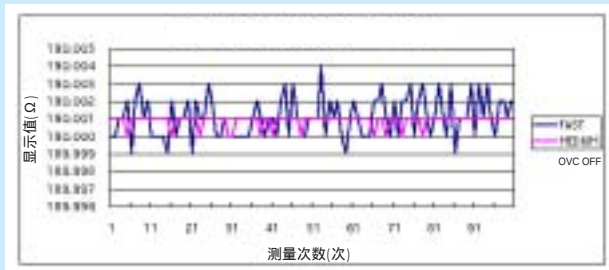
[200 Ω 量程/快·中]
