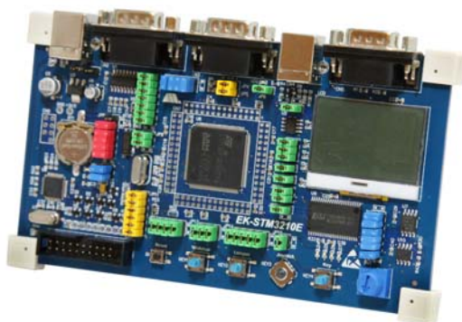
图 1: EK-STM3210E 照片
