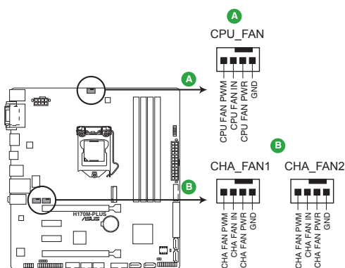
H170M-PLUS Fan connectors
