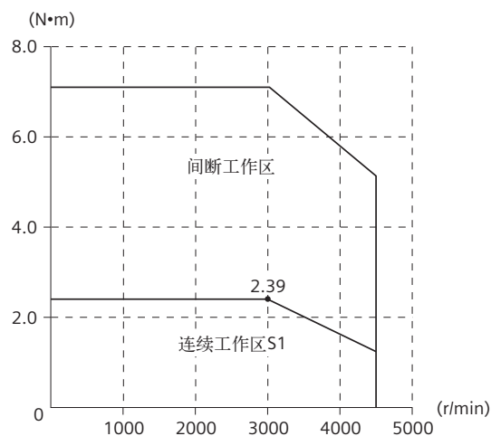
1FL4044-0AF21-.... (750W)
