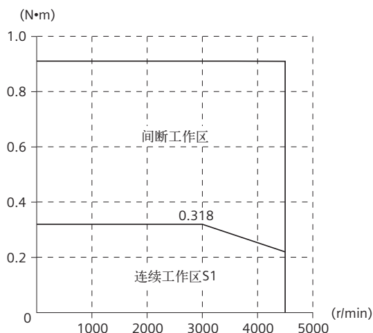
1FL4021-0AF21-.... (100W)
