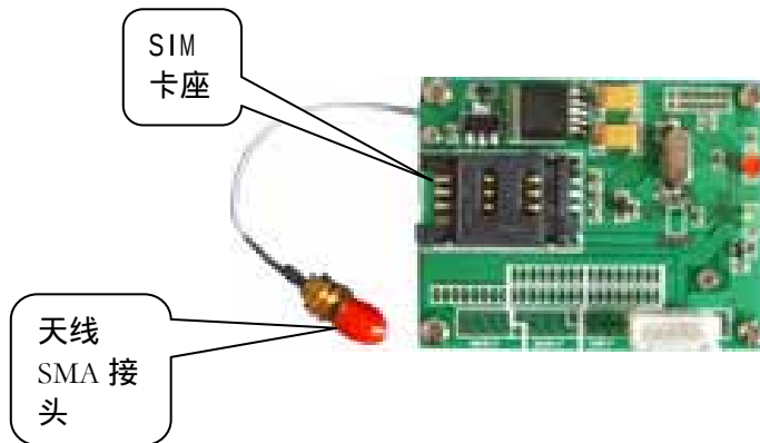
DTP-T09B 外型图片
