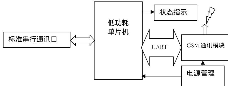
图 1. DTP-T09 系列 GSM 无线通信模块框图
