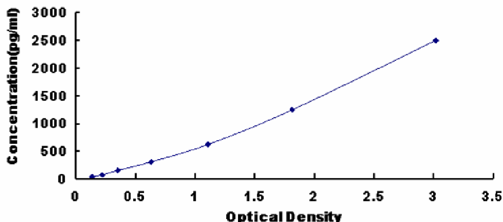
图 1: 小鼠肾损伤分子 1(Kim1)试剂盒标准曲线
