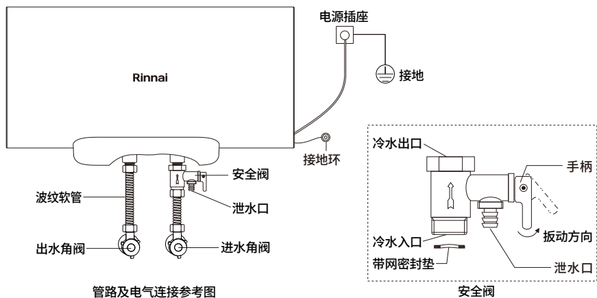
管路及电气连接参考图
