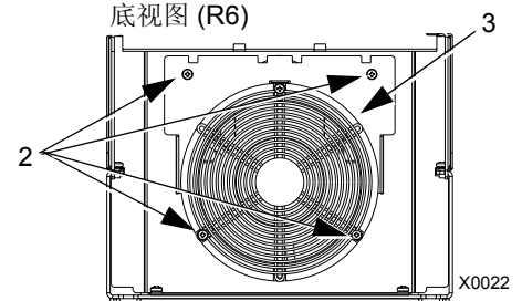
底视图 (R6)
