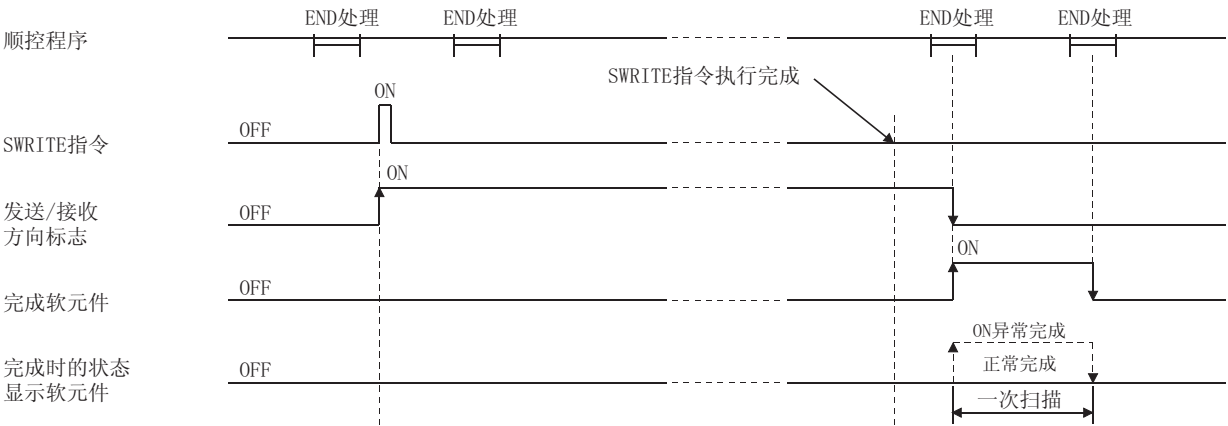
[正在执行 SWRITE 指令时其它站的运行]
