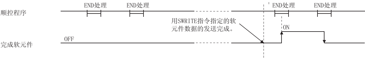
[正在执行 SWRITE 指令时其它站的运行]
