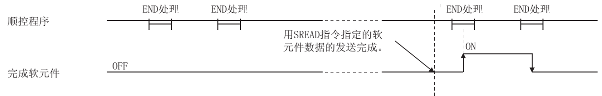
[正在执行 SREAD 指令时的其它站的运行]
