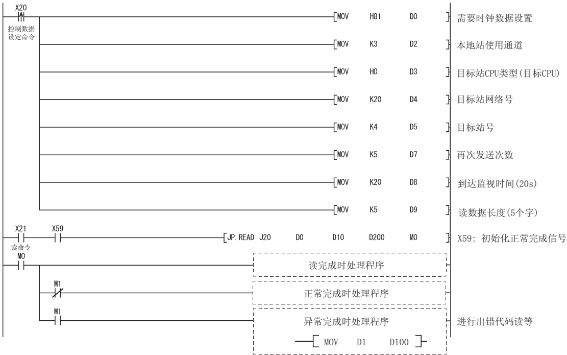
(a) 1 号站程序 (READ 指令) 当以太网模块的 I/O 信号是 X/Y40 至 X/Y5F 时
