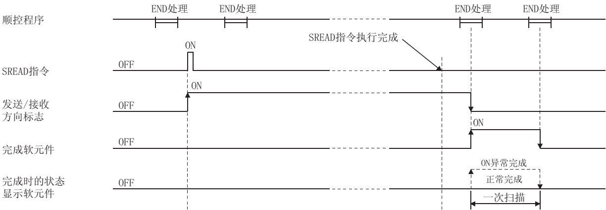
[正在执行 SREAD 指令时的其它站的运行]
