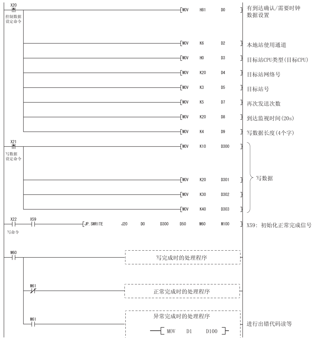
(b) 2 号站程序 (SWRITE 指令) 当以太网模块的 I/O 信号是 X/Y40 至 X/Y5F 时
