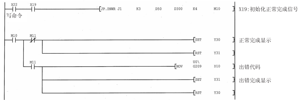
(b) 2 号站的程序 (ZNWR 指令)
