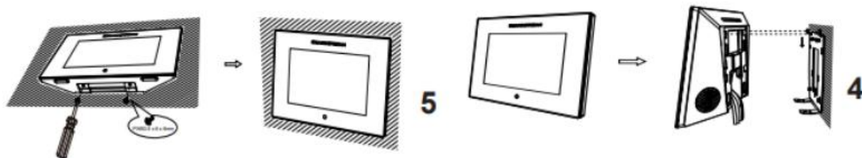
图 3 壁挂式安装
