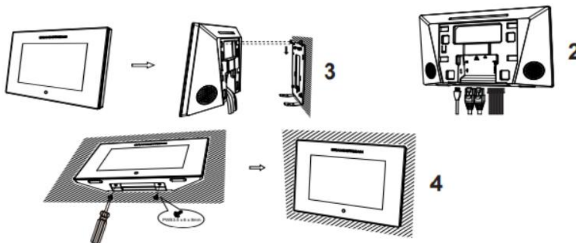
图 4 入墙式安装
