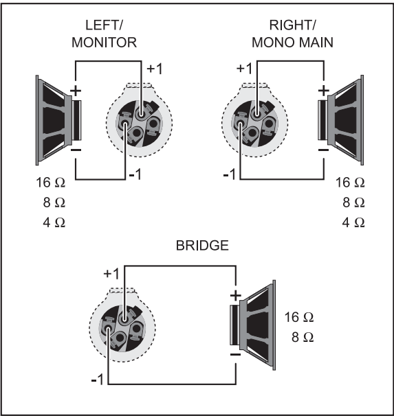
图 3.6: Speakon® 插头 Pin 配置
