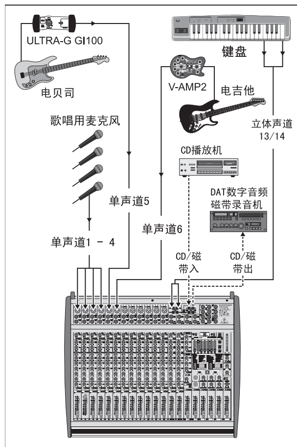
图 4.4: 标准设置 (举例)
