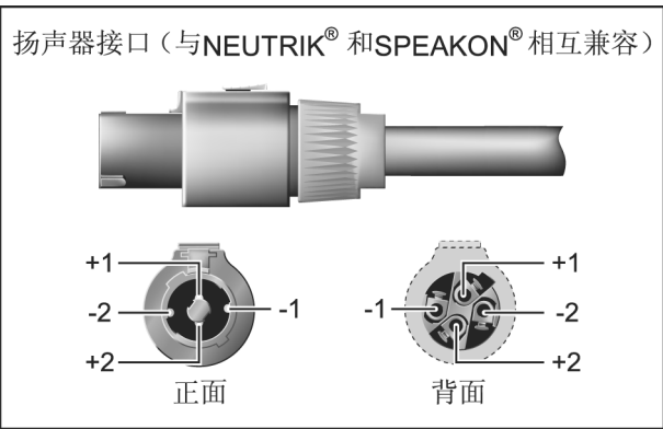
3.5: 专业扬声器接口
