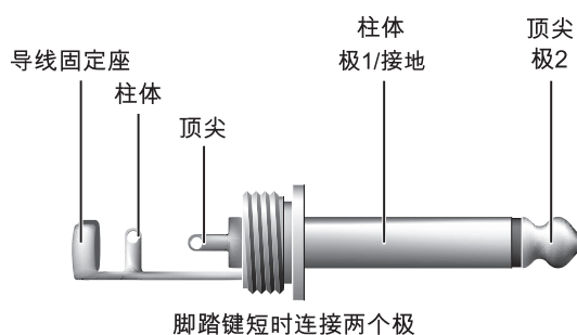
图 3. 4: 脚踏键的单声道插头
