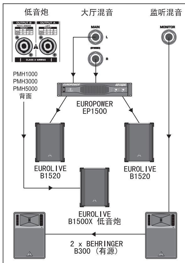
图 4.2: 单声道桥接运行
