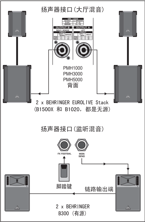
图 4.1: EUROPOWER 调音台作为立体声放大器
