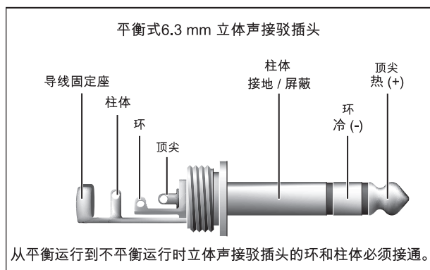
图 3. 2: 6.3mm 立体声道插头
