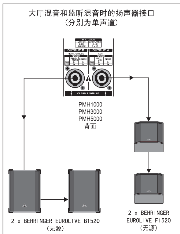
图 4.3: EUROPOWER 调音台作为单声双通道放大器 (举例)
