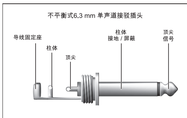
图 3. 1: 6.3mm 单声道插头
