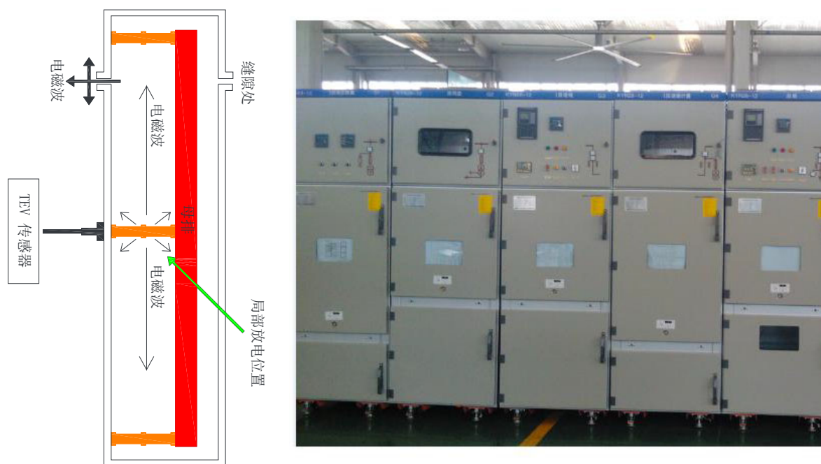
图 3-1 TEV 检测原理图
