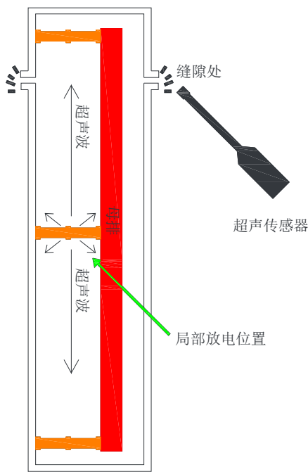
图 3-2 US 测量原理图
