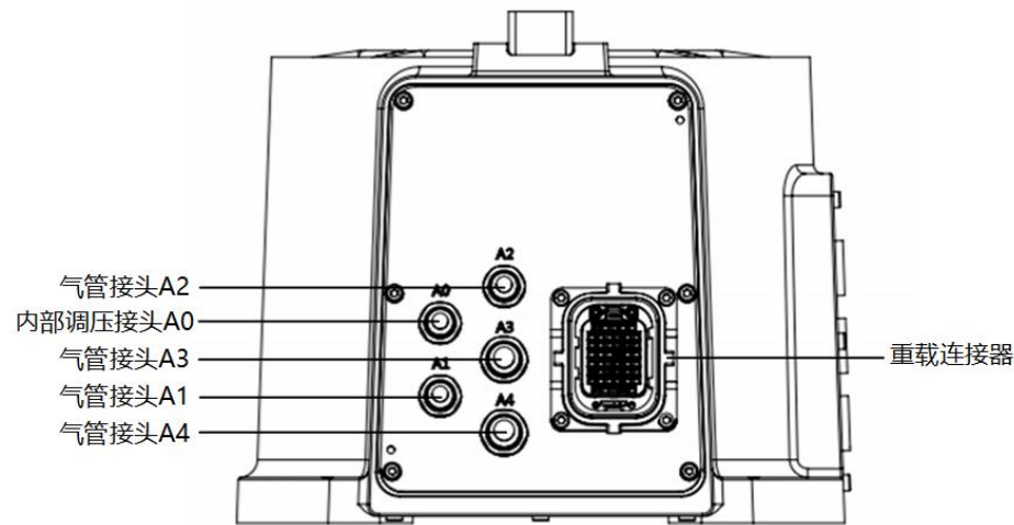
(a) 后视图
