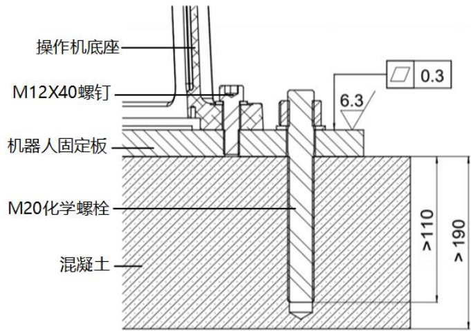
(b) 剖面图
