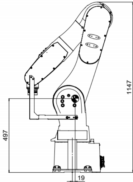
(a) 右视图
