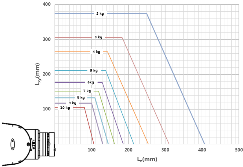
(b) 负载质心位置允许范围示意图
