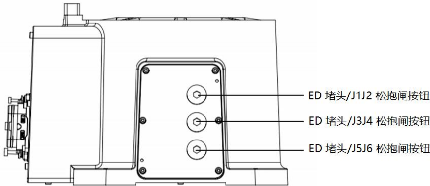
(b) 左视图
