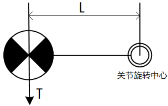
图 7-5 负载离心率示意图
