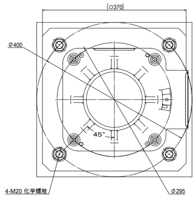
(a) 平面布置尺寸
