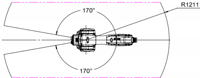
(b)俯视图
