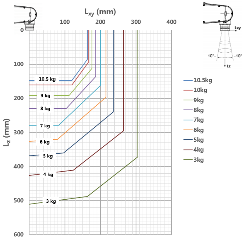
图 7-7 操作机腕部向下时的负载质心位置示意图
