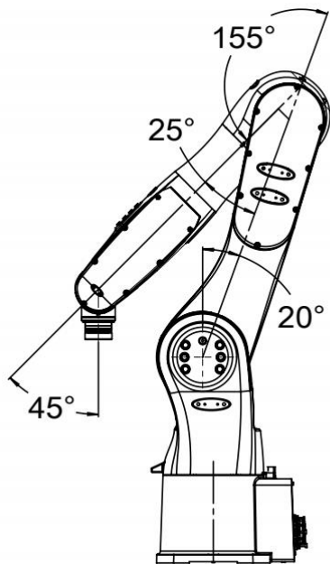
图 9-2 操作机搬运位姿图
