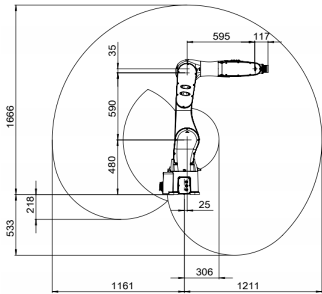
(a)侧视图
