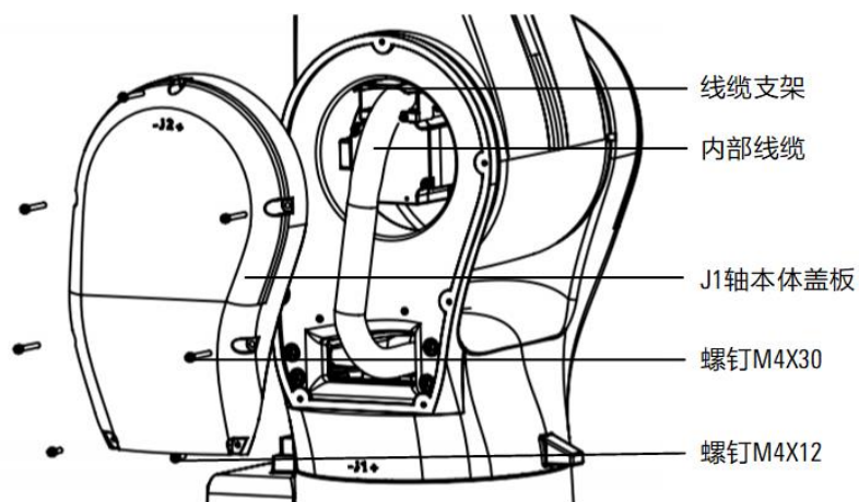
图 12-2 肩部内部线缆检修
