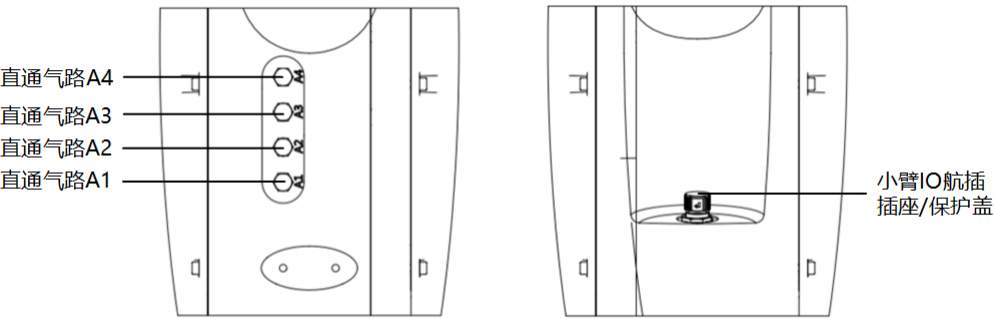
图 5-2 操作机小臂上接口
