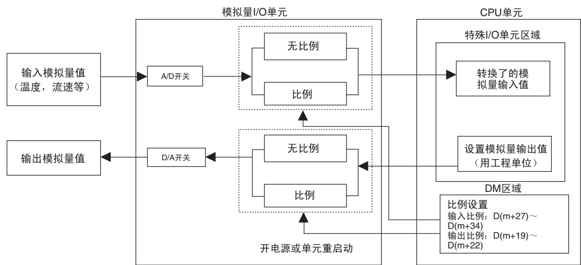
比例的概念图（仅对 CJ1W-MAD42）
