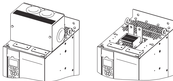
图 2.22 加盖（左）和未加盖（右）的负载共享或再生端子
