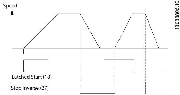
图 6.2 自锁启动/停止反逻辑
