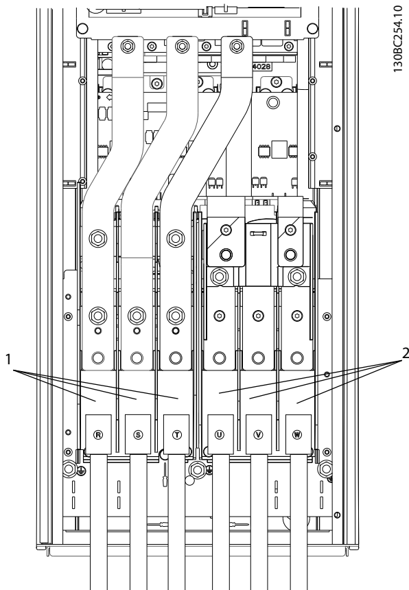
图 2.13 连接到交流主电源
