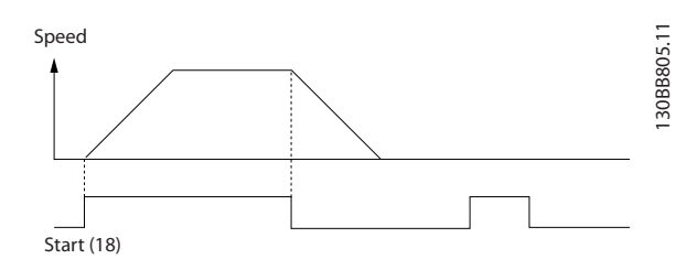
图 6.1 带安全停止功能的启动/停止命令
