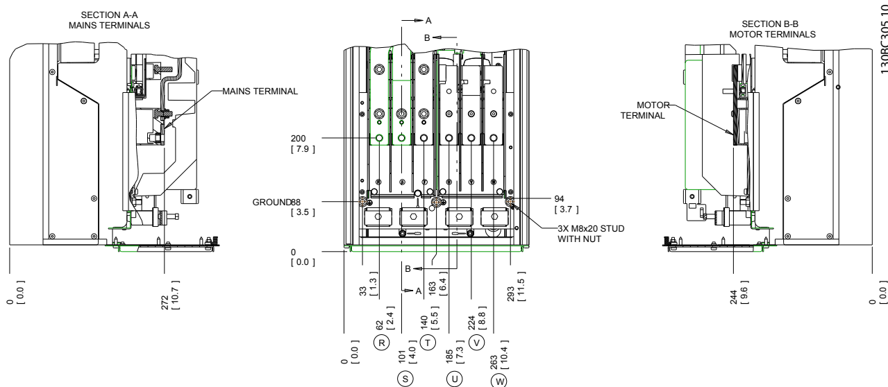
图 2.7 端子位置 D1h
