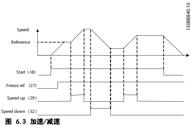
图 6.3 加速/减速
