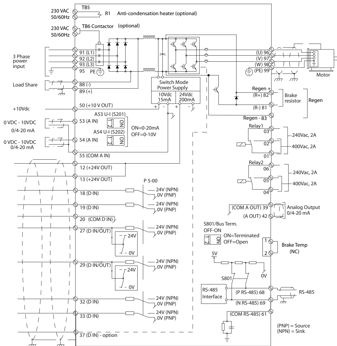
图 2.2 互连图
