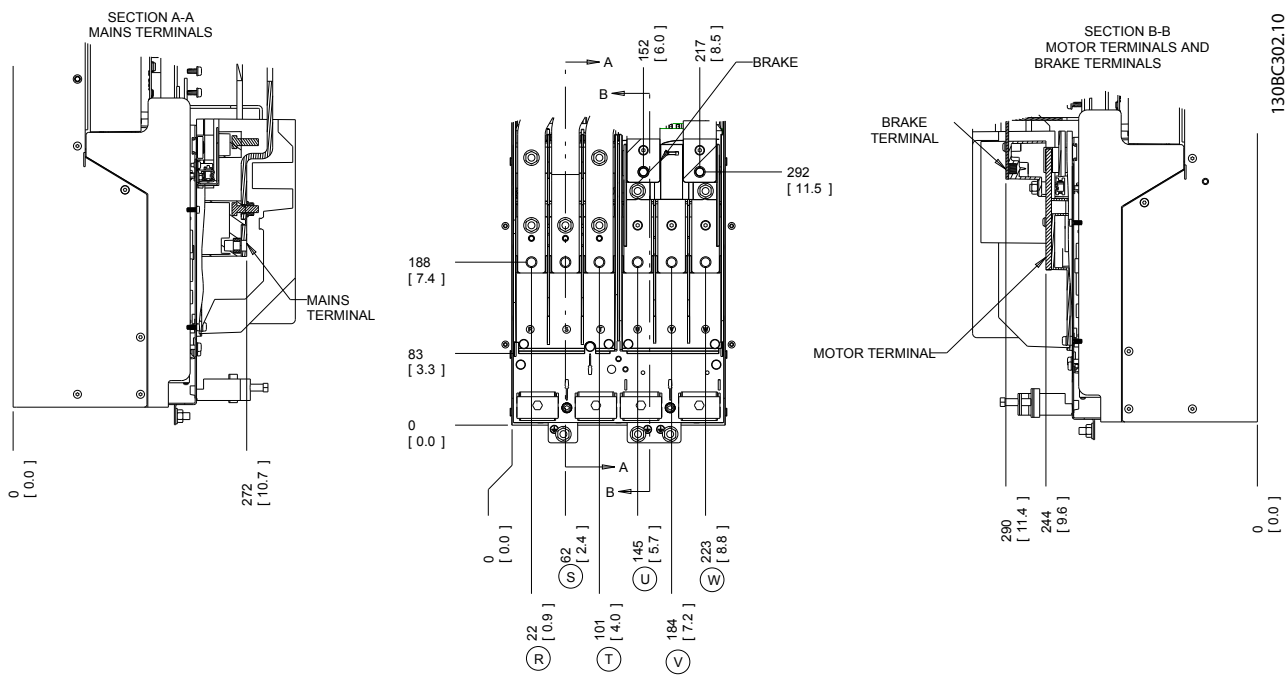
图 2.8 端子位置 D3h
