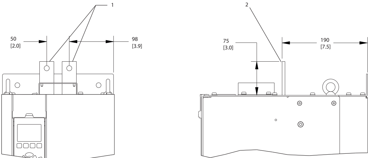
图 2.9 负载共享或再生端子, D3h
