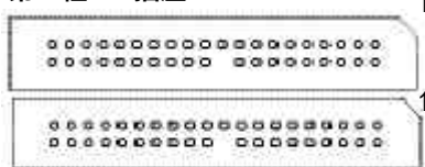
第一組 IDE 插座
