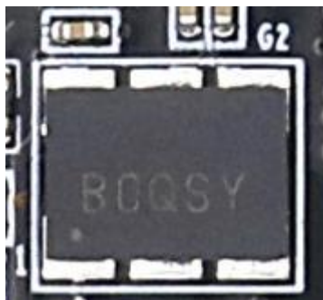
图 2-3-4 125M 有源晶振实物图
