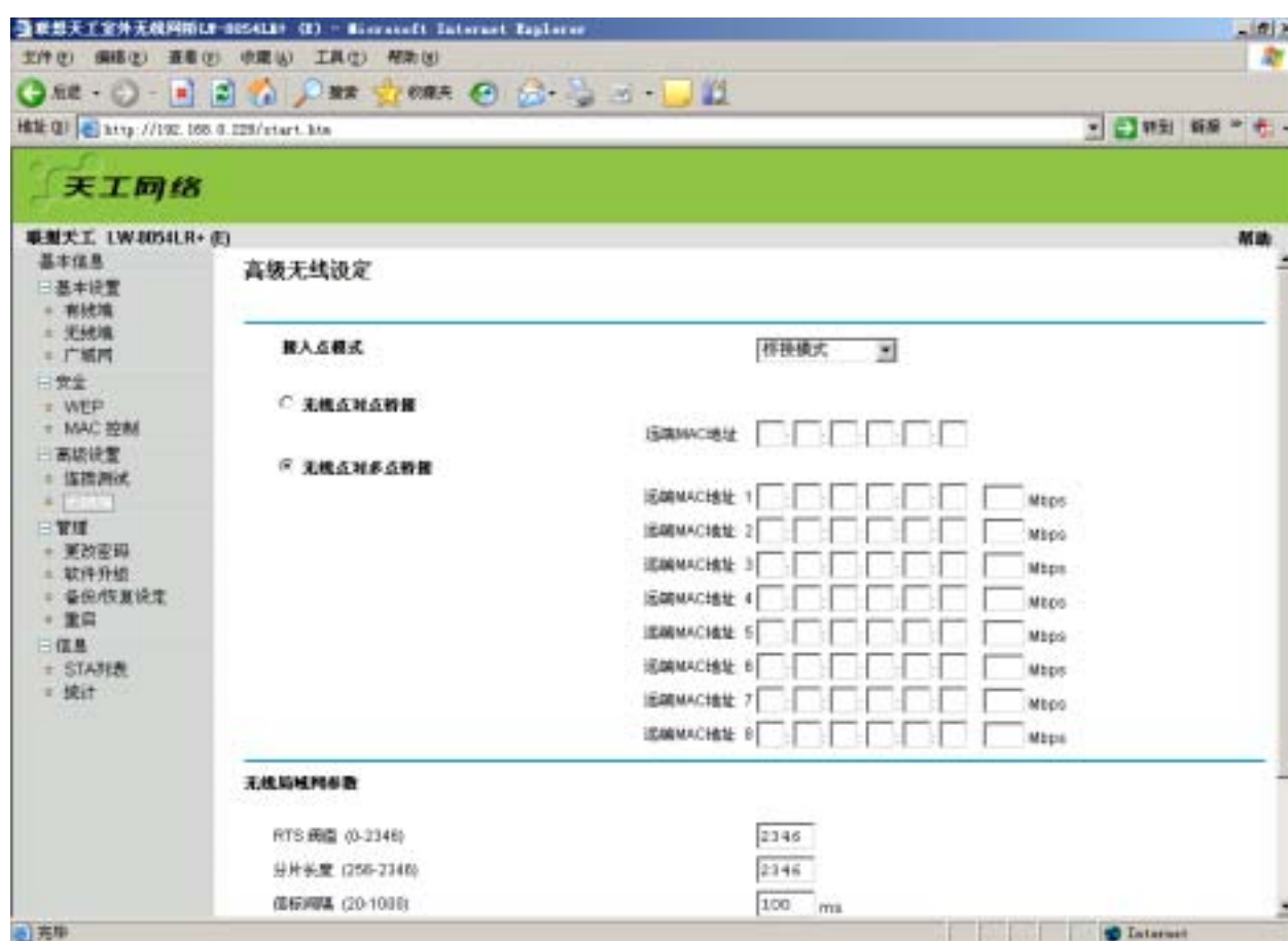
图 9 无线端配置
