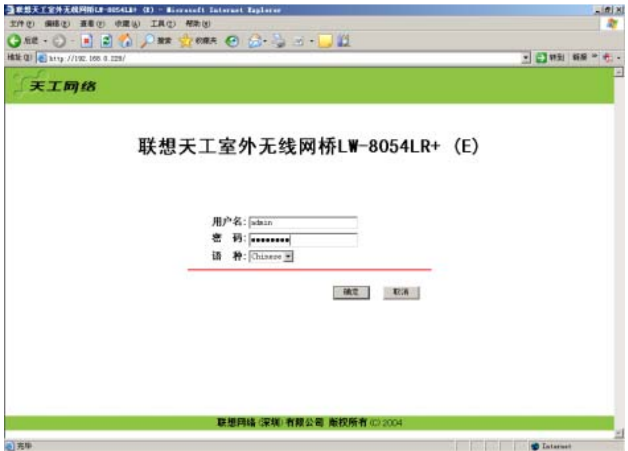
图 1 登录
