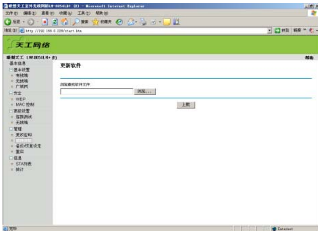
图 111 软件升级
