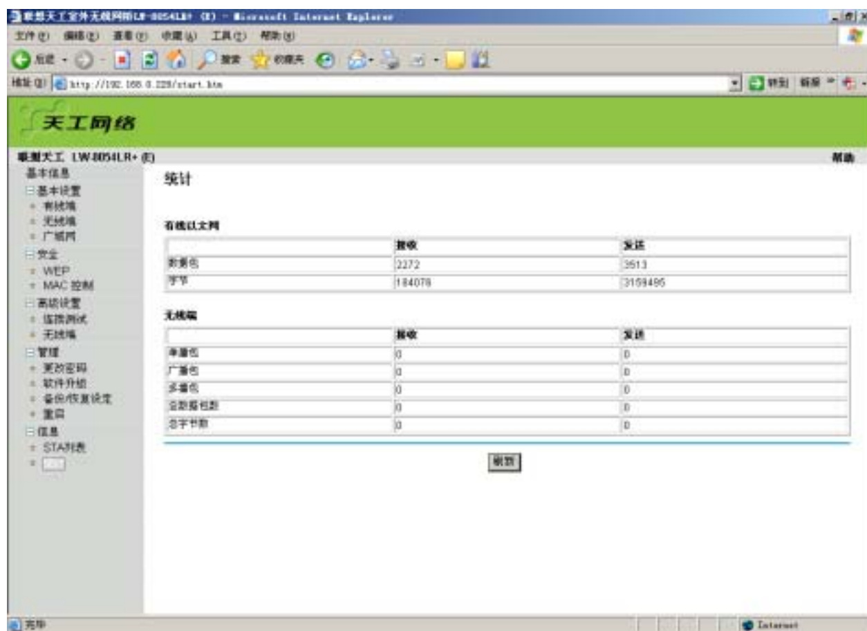
图 155 统计
