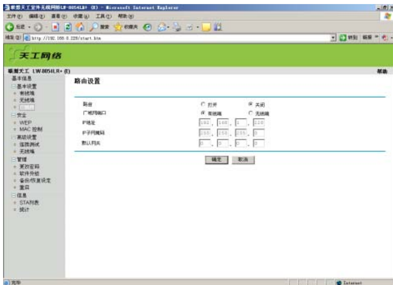
图 5 广域网配置
