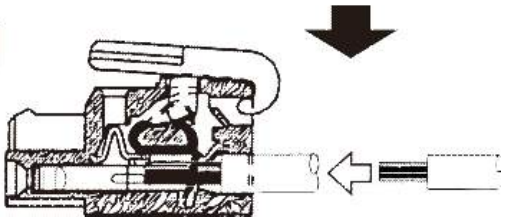
3) 按住接线杆将电缆朝箭头方向插入。
