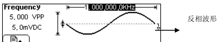
图 2- 81 反相波形
