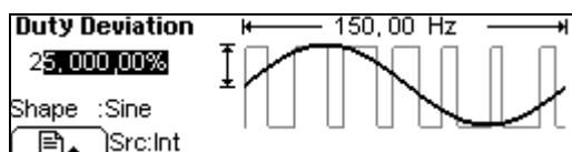
图 3- 11 输出PWM调制波形
