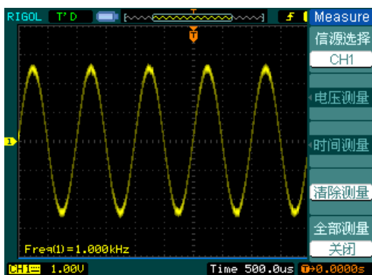
图 2- 69 DS1000中显示的波形
