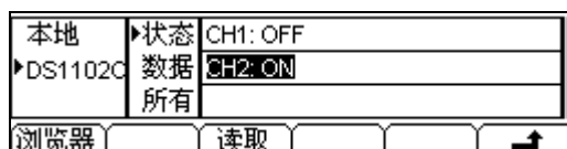
图 2- 66 选择信号源
