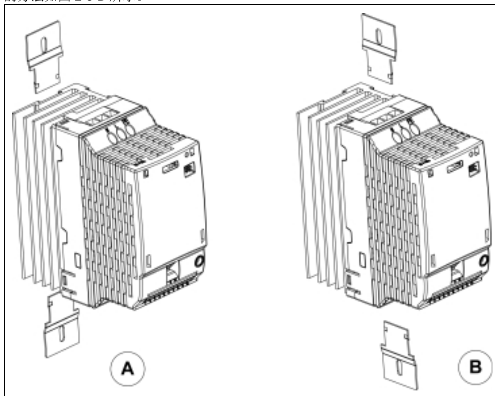
图 2-6 安装支架
