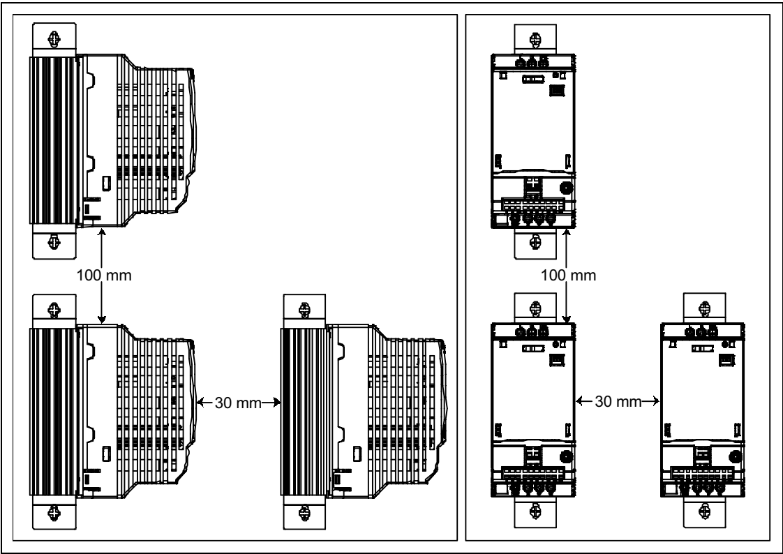
图 2-5 MICROMASTER 410 变频器间的安装间隙
