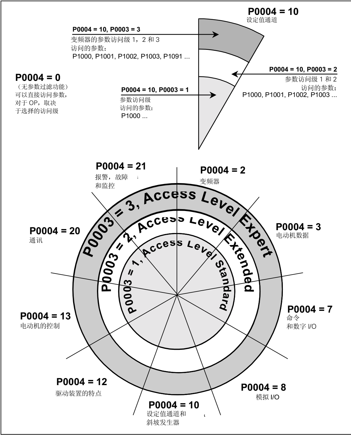
图 5-1 参数概览
