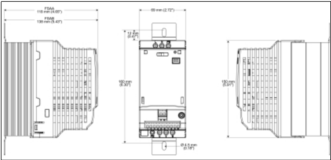
图 2-4 MICROMASTER 410 变频器的外形尺寸
