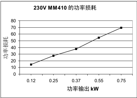
图 2-2 功率损耗，230 V
