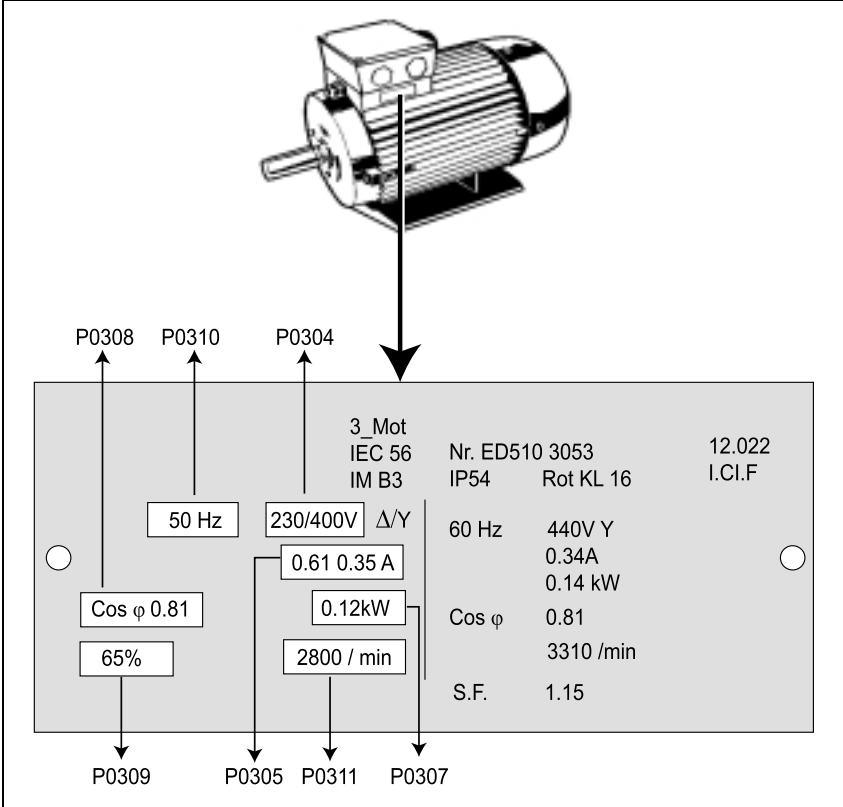
图 3-7 典型的电动机铭牌举例
