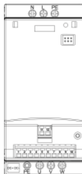
图 2-8 MICROMASTER 410 变频器的接线端子
