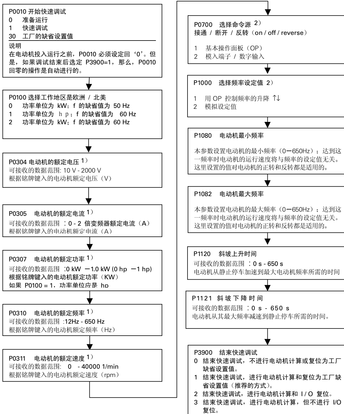
快速调试的流程图 (仅指第1访问级)
