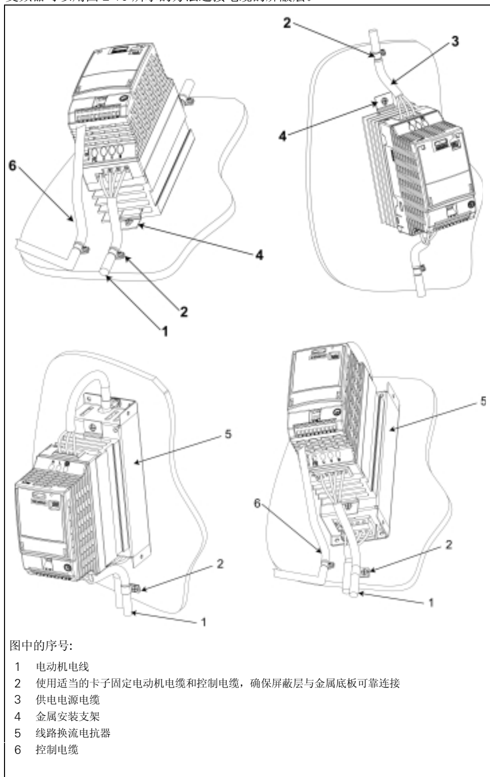
图 2-10 把电磁干扰（EMI）影响降到最小的布线方法
