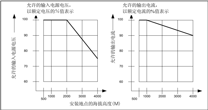
图 2-3 安装地点的海拔高度与额定参数的降格
