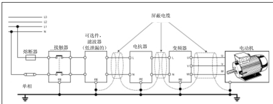
图 2-9 电动机和电源的接线方法
