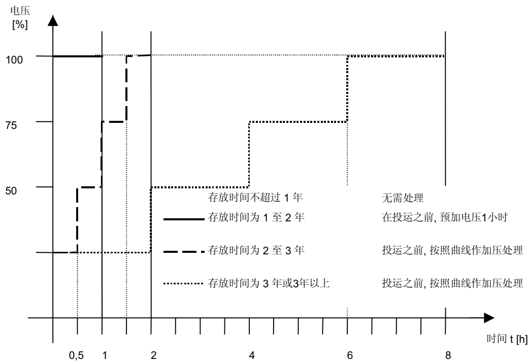
图 2-1 长期存放后投运前变频器的处理
