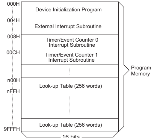
程序存储器
