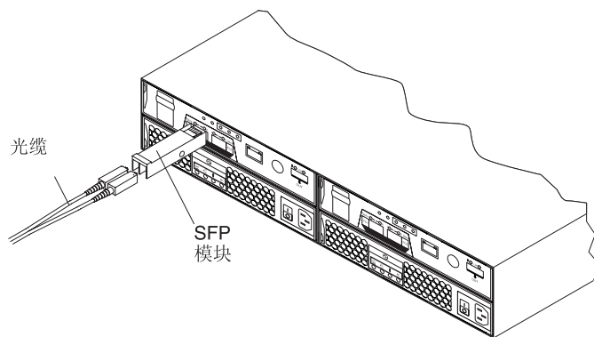
图 73. 更换 SFP 模块
