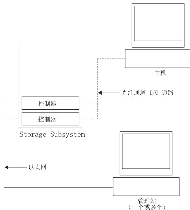
图 37. 直接（频带外）管理 Storage Subsystem
