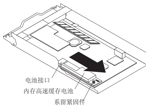
图 69. 从控制器中卸下电池
