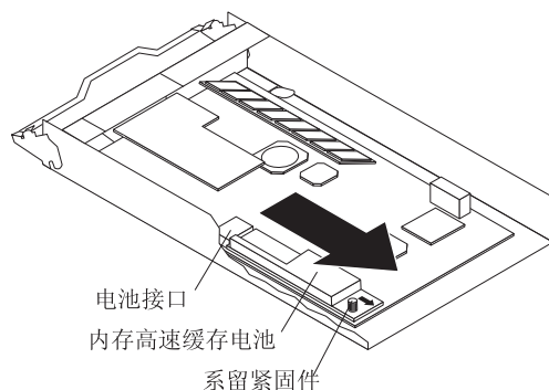
图 66. 从控制器中卸下并更换电池部件
