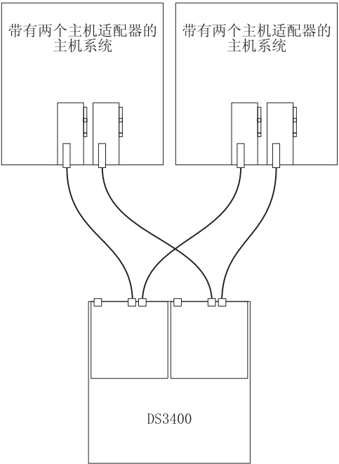
图 43. 到多主机中多 HBA 的双控制器直接连接的连接
