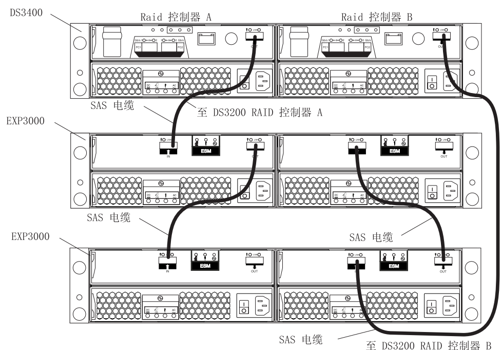
图 33. 一个双控制器 DS3400 和两个存储扩展箱
