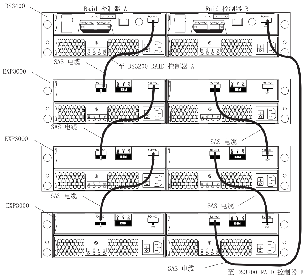
图 34. 一个双控制器 DS3400 和三个存储扩展箱
