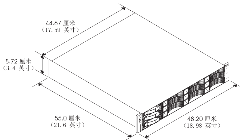
图 9. DS3400 尺寸
