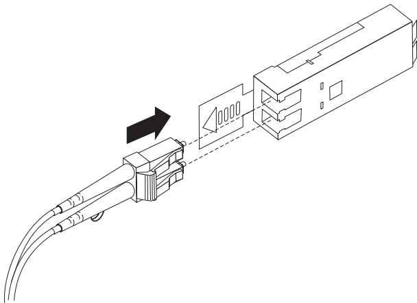
图 8. SFP 模块和光缆
