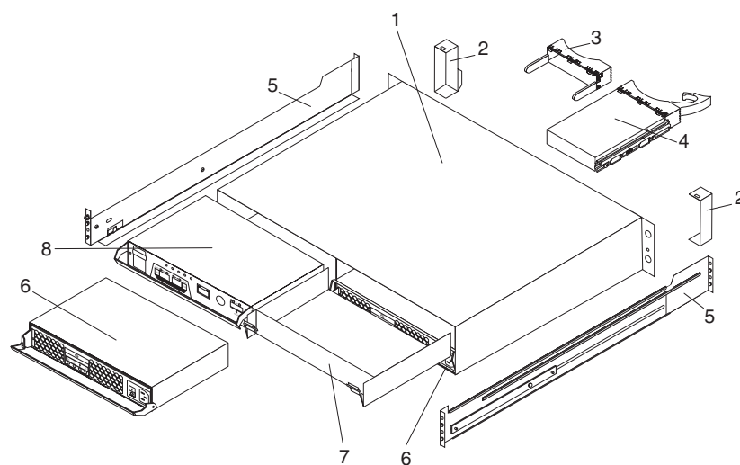
图 74. DS3400 Storage Subsystem 部件
