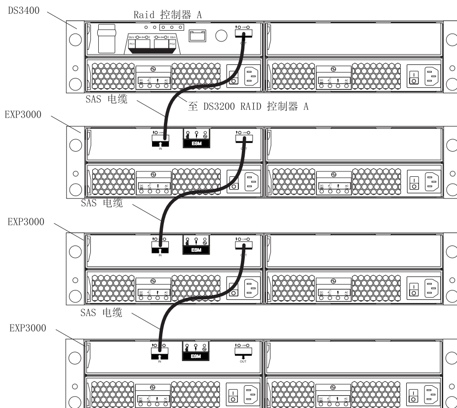
图 31. 一个单控制器 DS3400 和多个单 ESM 存储扩展箱
