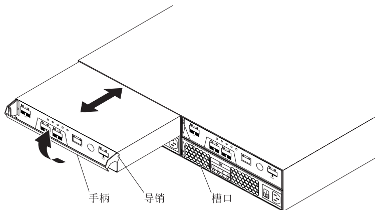
图 68. 卸下控制器
