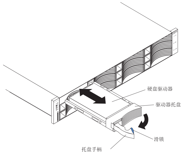
图 63. 安装和卸下硬盘驱动器
