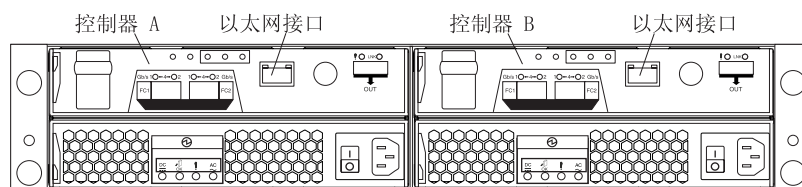
图 35. 双控制器 DS3400 上以太网端口的位置
