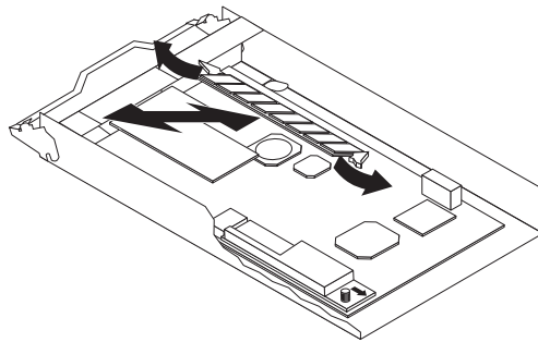
图 71. 将 DIMM 安装到控制器上
