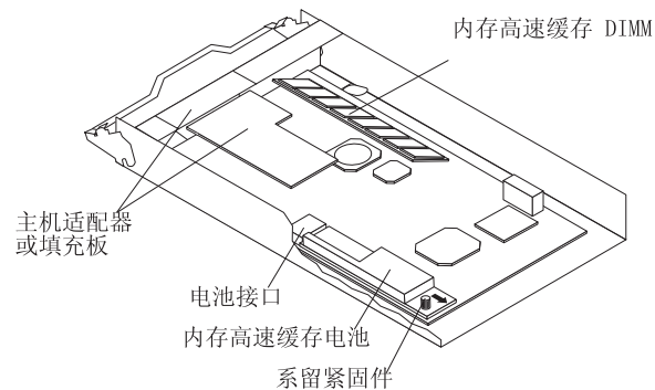
图 67. 内存高速缓存 DIMM 的位置
