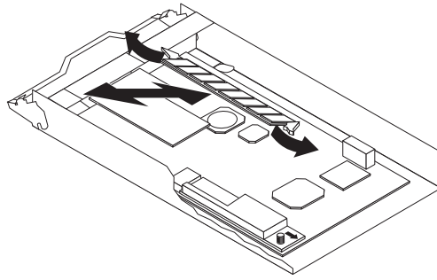
图 70. 从接口中卸下 DIMM
