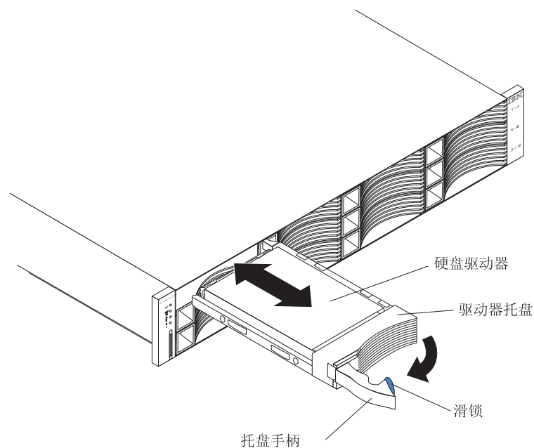
图 62. 卸下驱动器
