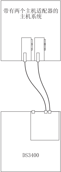
图 40. 到双 HBA 的单控制器直接连接的连接（冗余主机连接）
