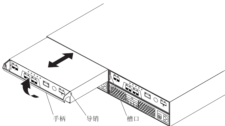
图 72. 重新安装控制器
