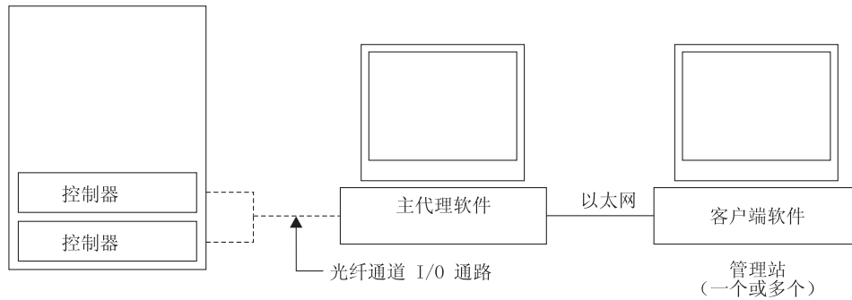
图 36. 主机代理（频带内）管理 Storage Subsystem
