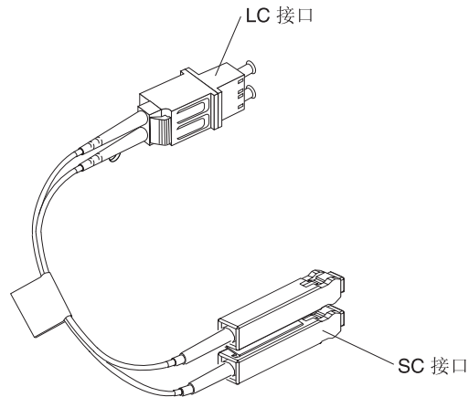
图 21. LC-SC 光纤通道电缆适配器
