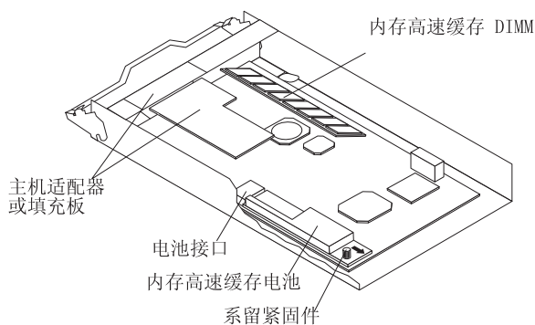
图 7. 电池部件
