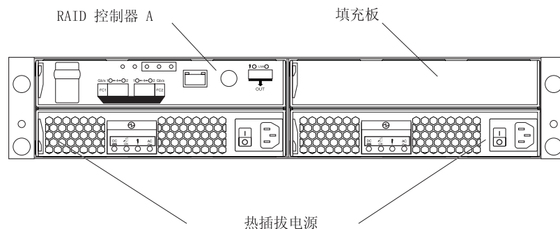
图 3. 单控制器型号的后视图
