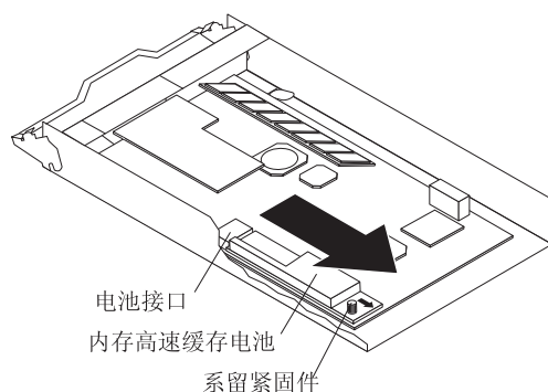
图 60. 从控制器中卸下电池
