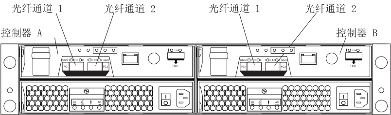
图 38. DS3400 上 RAID 控制器的主机接口位置
