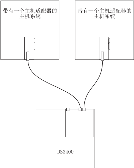
图 41. 到多主机中单 HBA 的单控制器直接连接的连接
