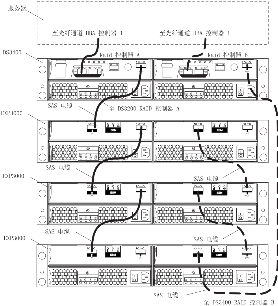
图 29. 冗余驱动器路径示例
