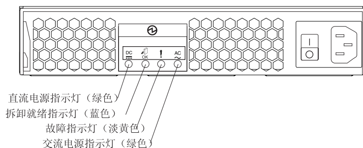
图 48. 电源指示灯
