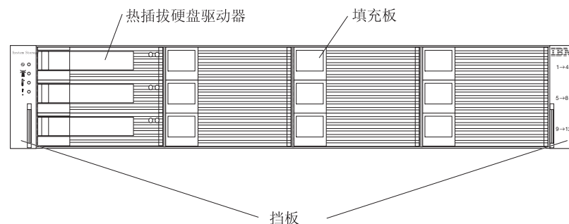
图 2. DS3400 热插拔驱动器托架
