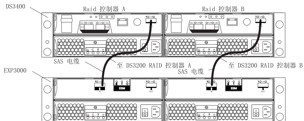
图 32. 一个双控制器 DS3400 和一个存储扩展箱
