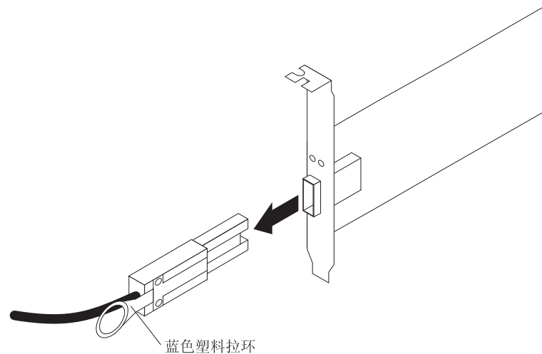
图 28. 拔出迷你 SAS 电缆
