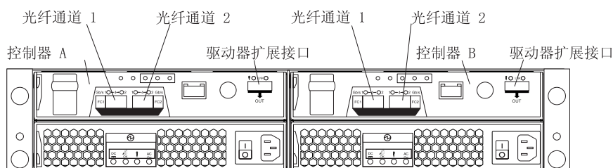
图 30. DS3400 Storage Subsystem 端口和控制器
