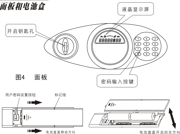
图5 电池盒的开启
