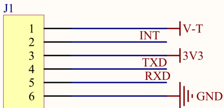
图 3-3 BFM530T 串口接口(J1)
