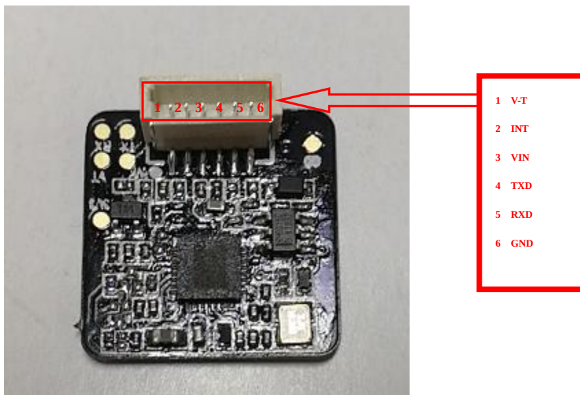
图 3-2 BFM530T 模块图反面
