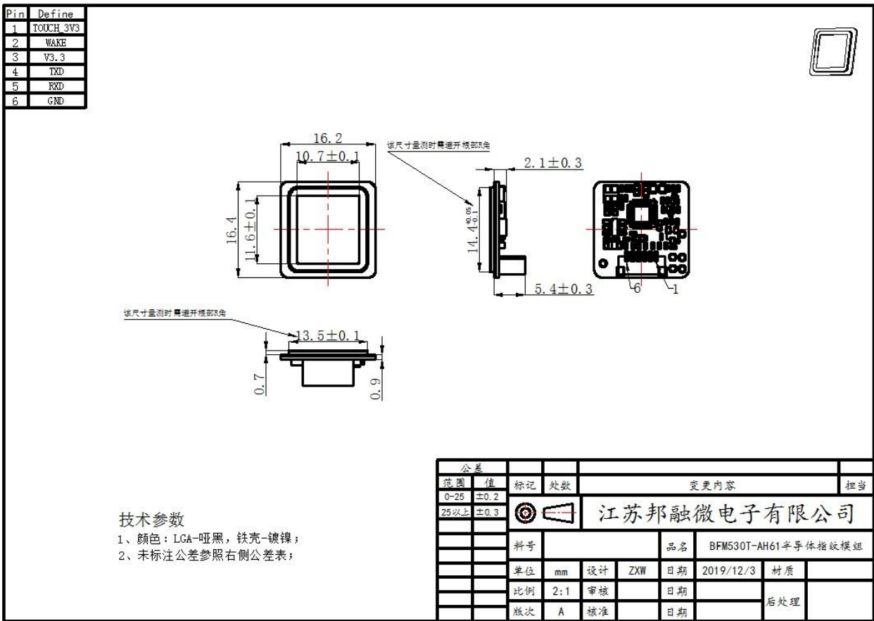
图 7-1 尺寸信息
