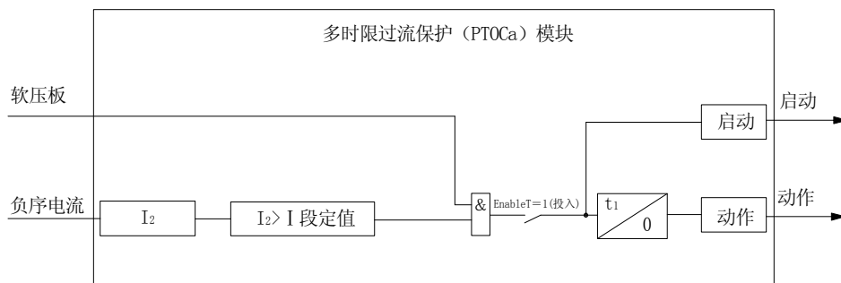
图4-6 负序过流I段保护原理框图
