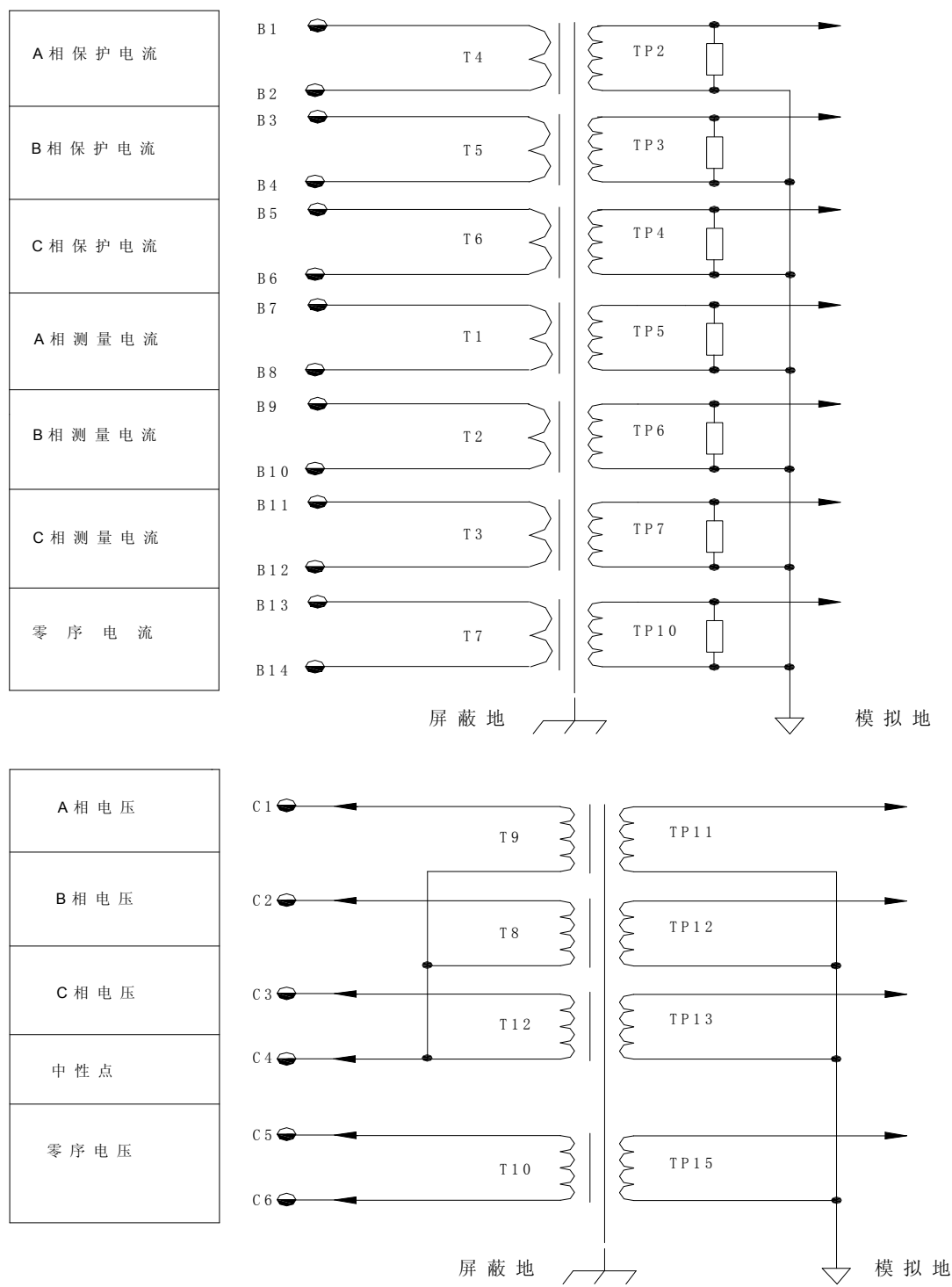
附图 1 DSI 5153 交流回路原理图
