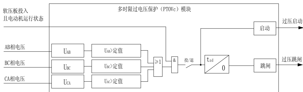
图4-12 过电压保护原理框图
