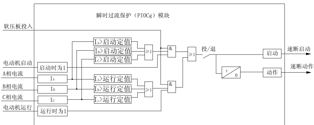
图4-4 速断保护原理框图（过流与速断同）
