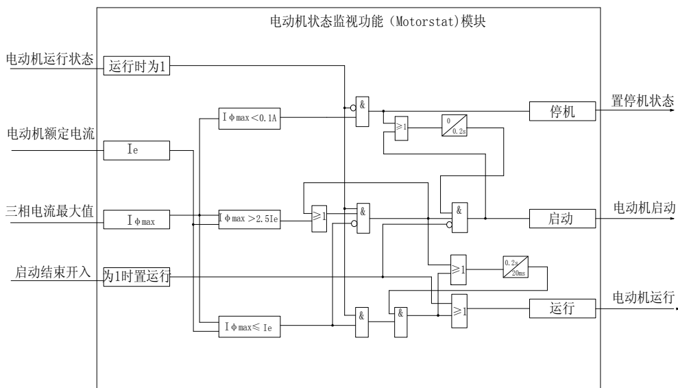
图4-2 电动机状态监视原理框图
