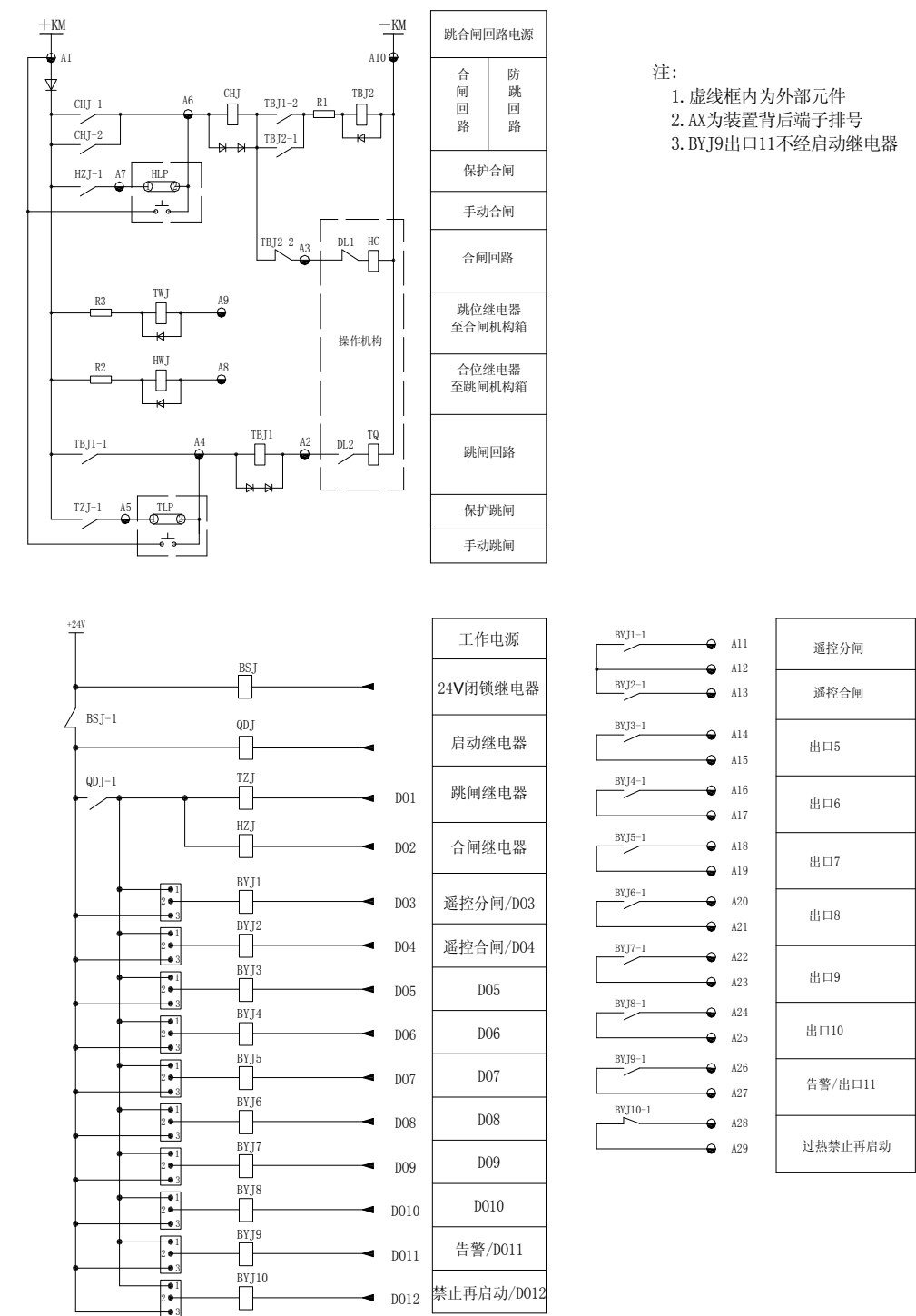
附图 2 DSI 5153 出口及操作回路原理图
