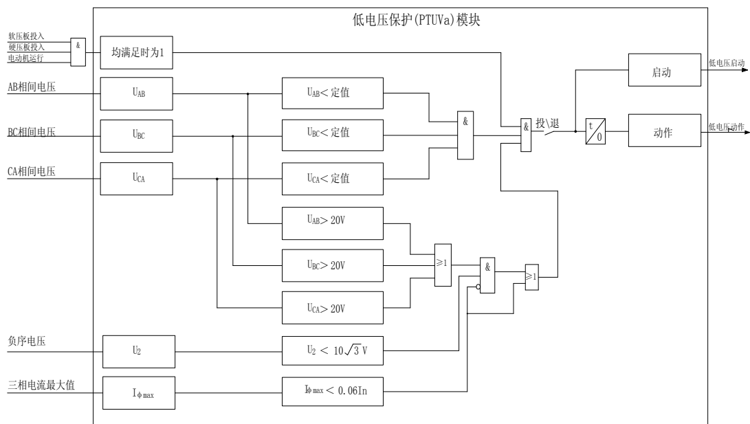
图4-13 低电压保护原理框图
