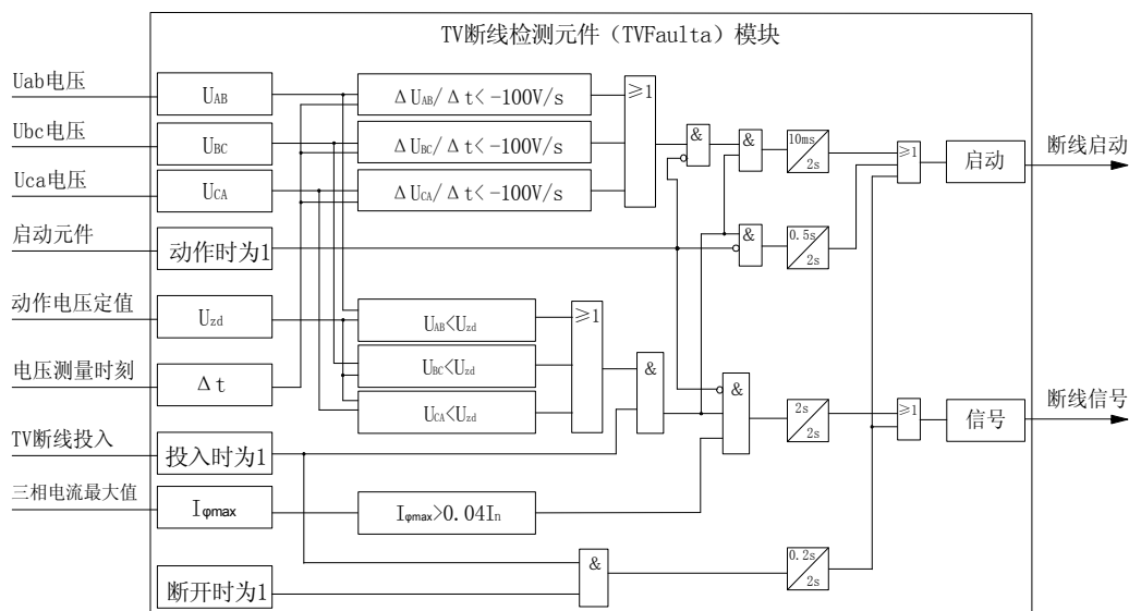
图4-15 TV断线检测元件原理框图
