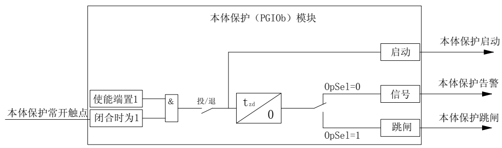
图4-18 本体保护原理框图
