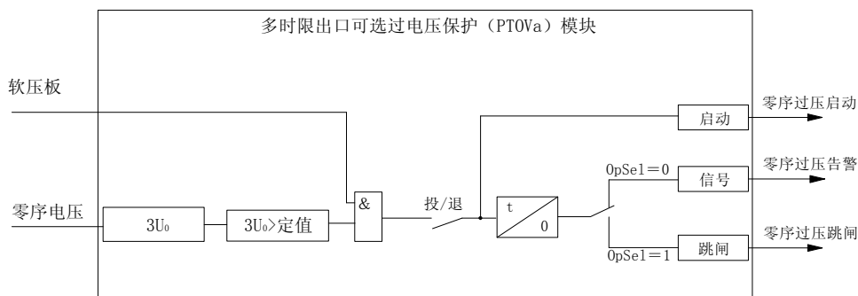
图4-10 零序过压保护原理框图
