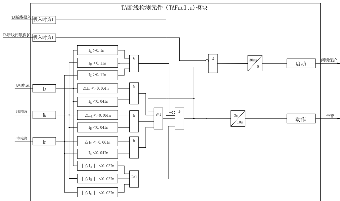
图4-16 TA断线检测元件原理框图
