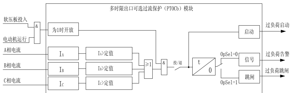
图4-11 过负荷保护原理框图
