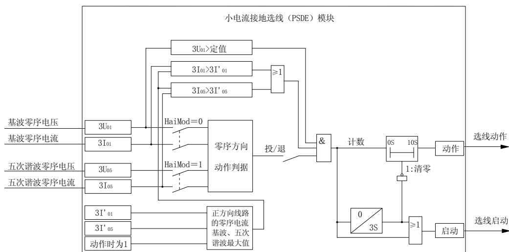
图4-9 小电流接地选线原理框图
