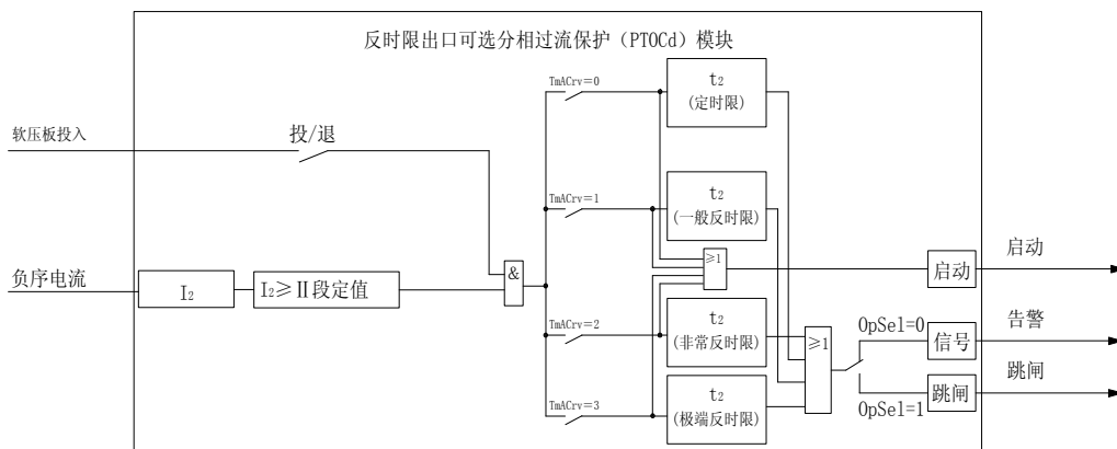
图4-7 负序过流II段保护原理框图
