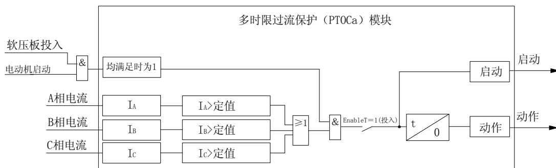
图4-3 启动时间过长保护原理框图
