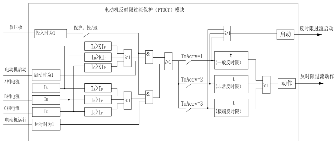
图4-5 反时限过流保护原理框图
