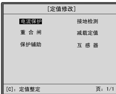
图5-8 定值修改菜单
