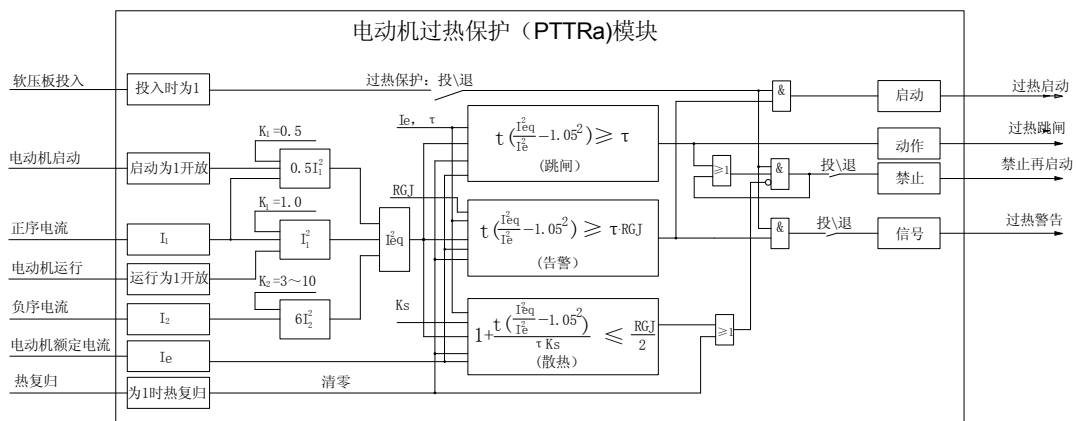
图4-14 电动机过热保护原理框图
