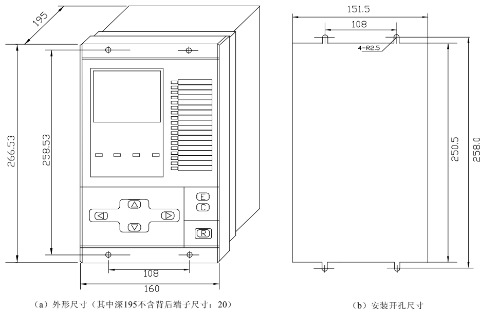
图 3—1 装置外形尺寸及安装开孔尺寸
