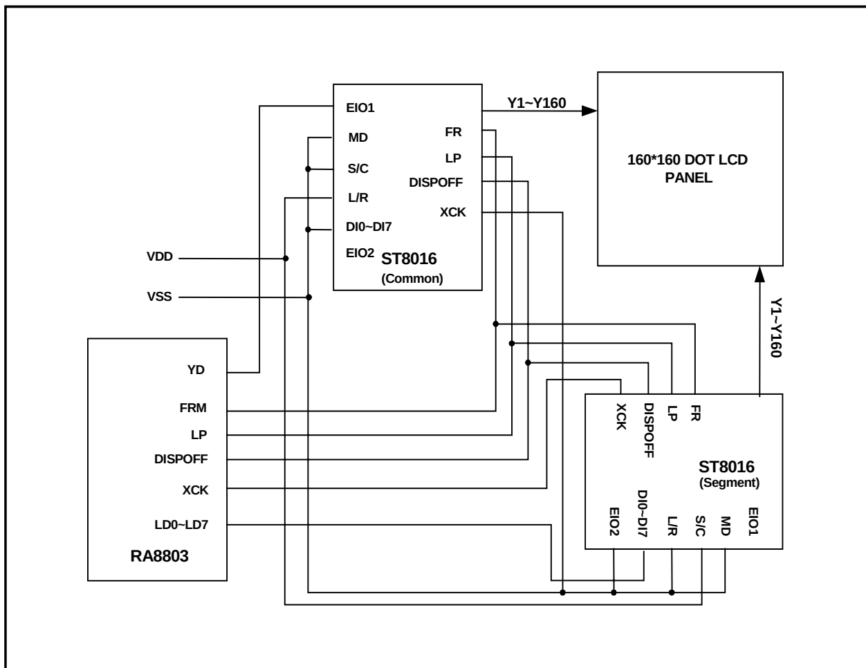
图 3-1：RA8803/8822 与 LCD Driver(ST8016)的接线图
