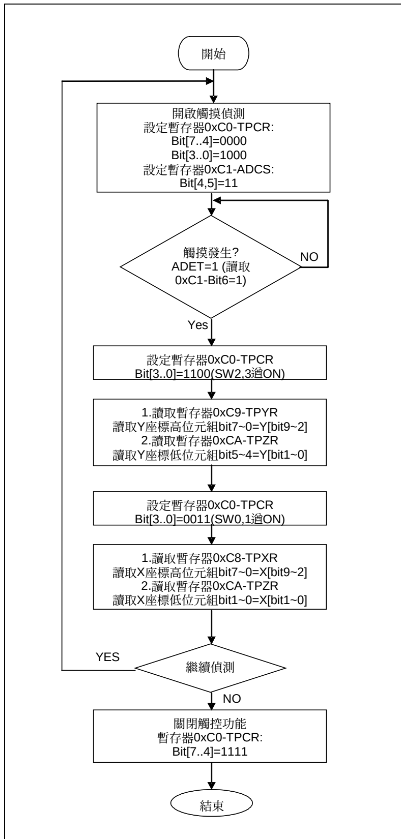
图 6-9：触摸式面板读取的控制流程图
