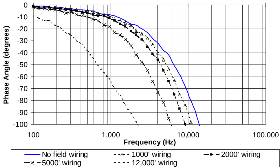
图 11 相位响应，典型 3300 XL 8 mm 5 m 系统带有各种长度的现场 联线，无安全栅
