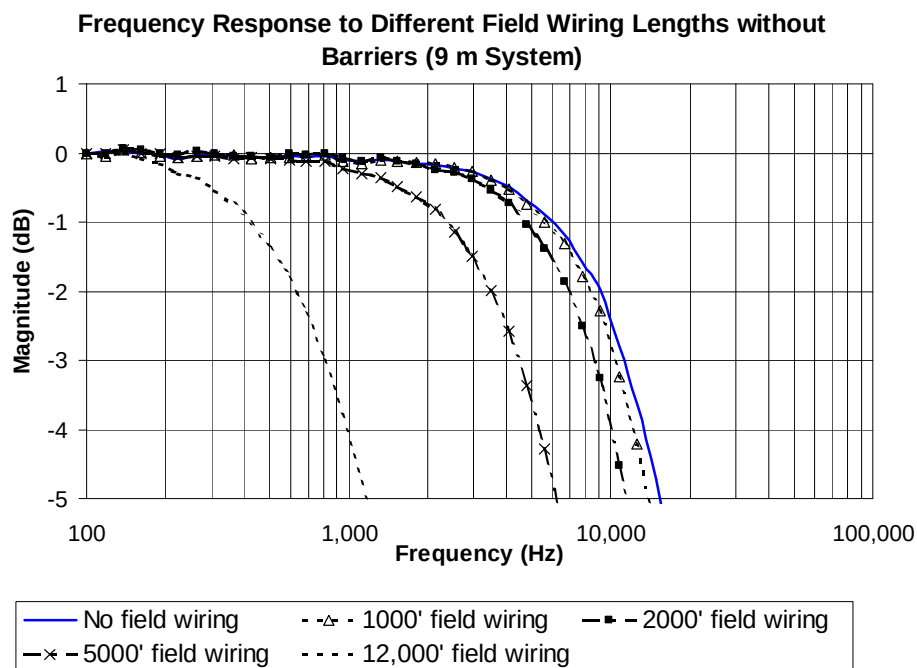
图 12 频率响应，典型 3300 XL 8 mm 9 m 系统带有各种长度的现场联线，无安全栅
