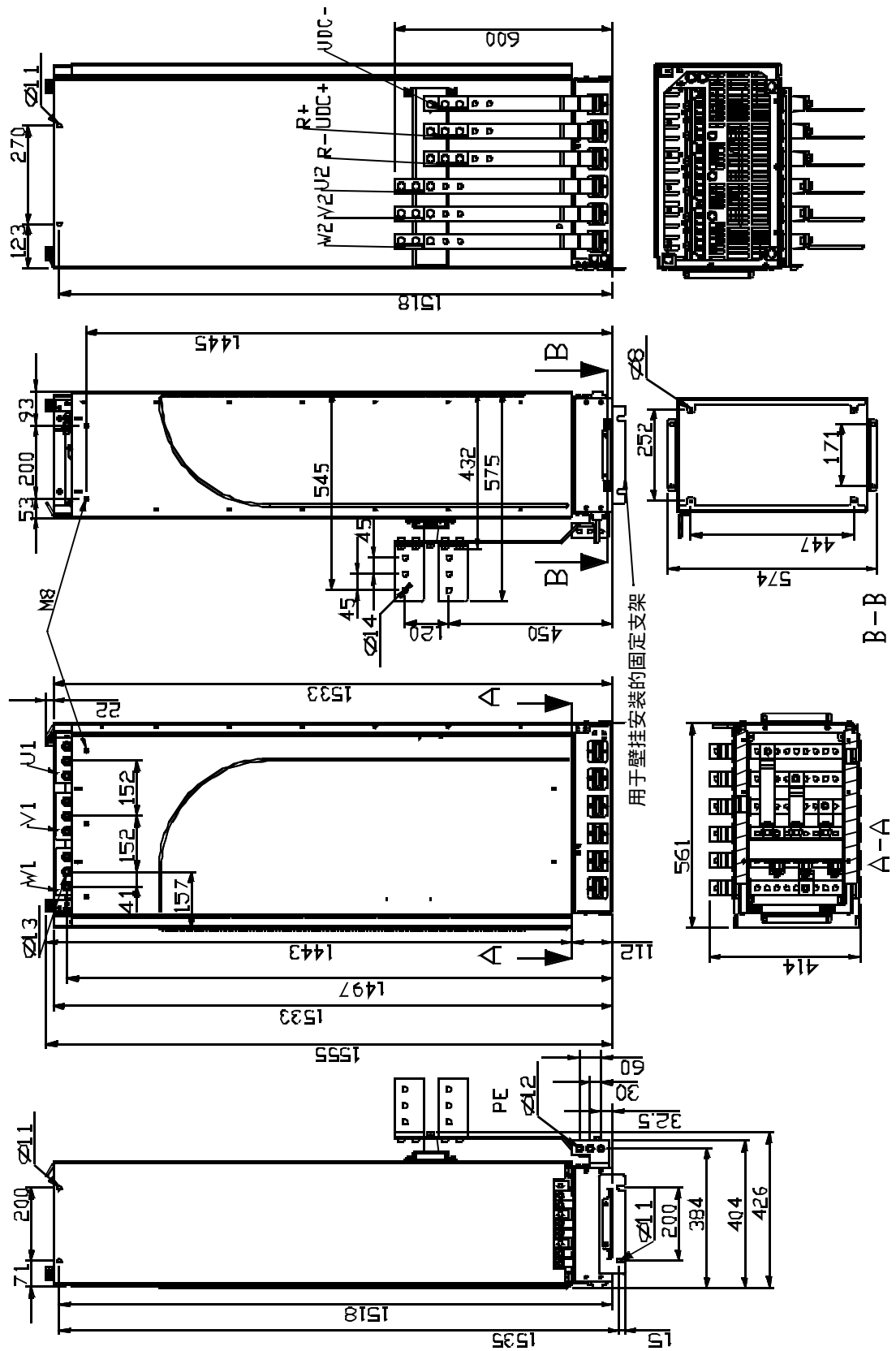
外形规格 R8 (mm)
