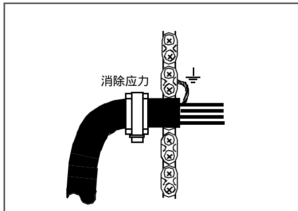
单屏蔽电缆
