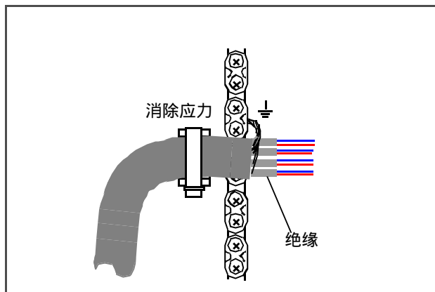
双屏蔽电缆
