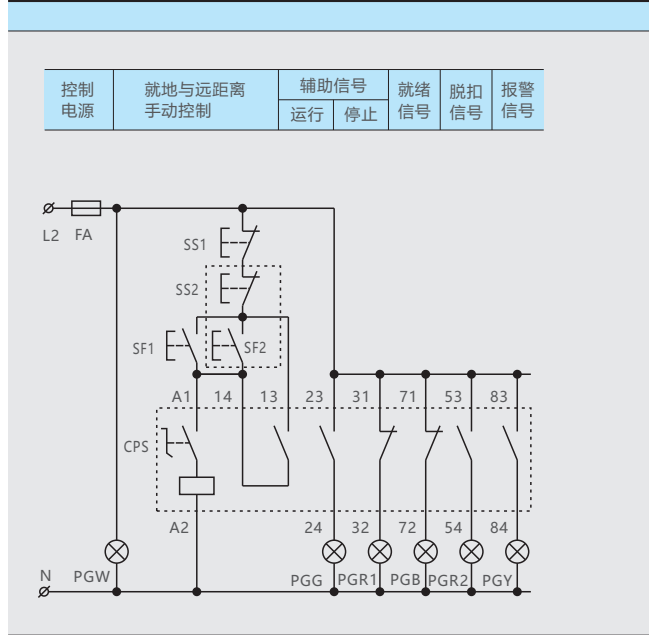
(4) 就地与远距离手动控制电路图
