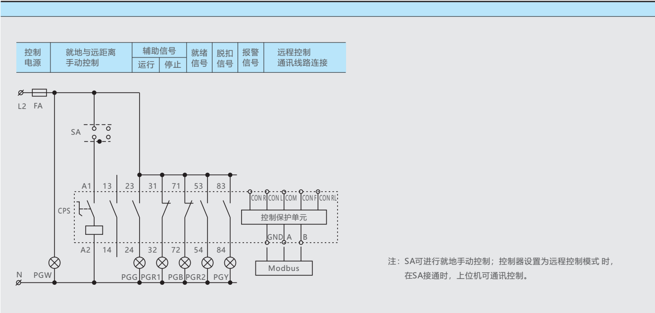
(5) 通讯远程控制电路图（配通讯型控制器）
