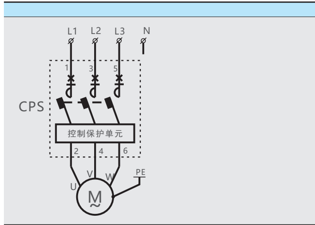
(4) 就地与远距离手动控制电路图
